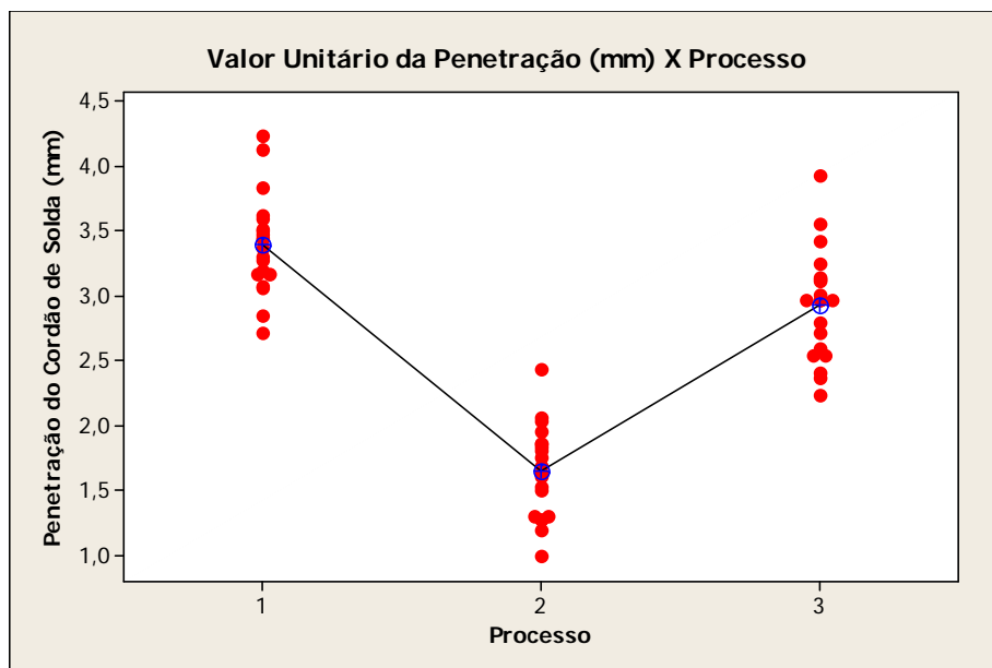
Figura 4. Comparação dos resultados das penetrações dos cordões de solda para cada processo. Fonte: TEIXEIRA, G.S. Análise da influência dos parâmetros de soldagem sobre a geometria do cordão de solda depositado pelo processo de soldagem TIG - MAG em tandem. Dissertação de mestrado. Universidade Federal do Rio Grande do Sul, Porto Alegre, 2011. (8)
