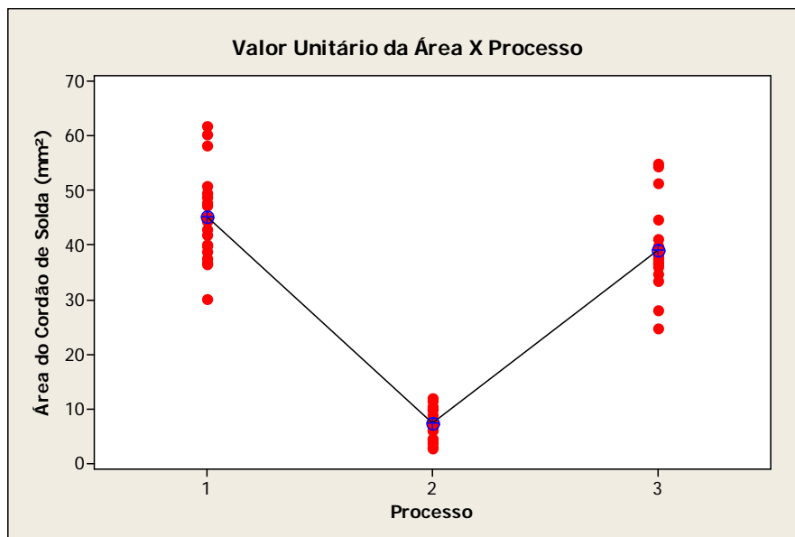
Figura 3. Comparação dos resultados das áreas dos cordões de solda para cada processo. Fonte: TEIXEIRA, G.S. Análise da influência dos parâmetros de soldagem sobre a geometria do cordão de solda depositado pelo processo de soldagem TIG - MAG em tandem. Dissertação de mestrado. Universidade Federal do Rio Grande do Sul, Porto Alegre, 2011. (8)
