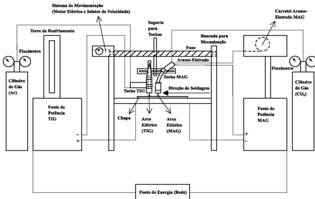
Figura 1. Esquema dos equipamentos utilizados na execução dos cordões de solda. Fonte: TEIXEIRA, G.S. Análise da influência dos parâmetros de soldagem sobre a geometria do cordão de solda depositado pelo processo de soldagem TIG - MAG em tandem. Dissertação de mestrado. Universidade Federal do Rio Grande do Sul, Porto Alegre, 2011. (8)
