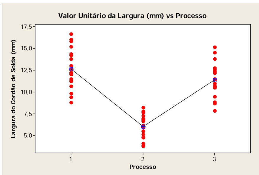
Figura 5. Comparação dos resultados das larguras dos cordões de solda para cada processo. Fonte: Fonte: TEIXEIRA, G.S. Análise da influência dos parâmetros de soldagem sobre a geometria do cordão de solda depositado pelo processo de soldagem TIG - MAG em tandem. Dissertação de mestrado. Universidade Federal do Rio Grande do Sul, Porto Alegre, 2011. (8)
