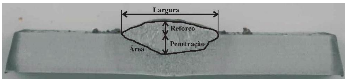
Figura 2. Dimensões do cordão de solda. Fonte: TEIXEIRA, G.S. Análise da influência dos parâmetros de soldagem sobre a geometria do cordão de solda depositado pelo processo de soldagem TIG - MAG em tandem. Dissertação de mestrado. Universidade Federal do Rio Grande do Sul, Porto Alegre, 2011. (8)
