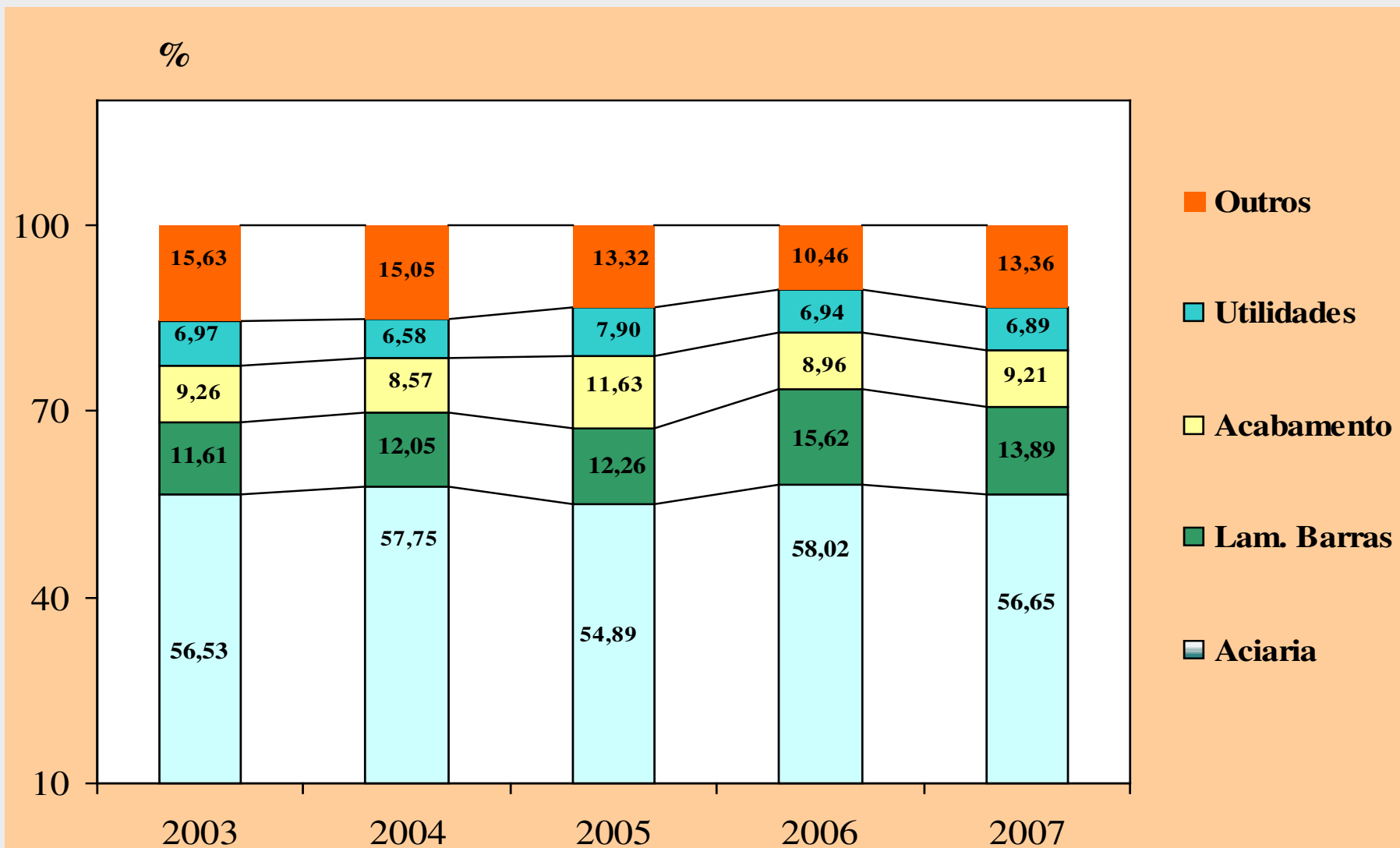
Fig. 2 - Evolução do Consumo de Energia Elétrica por Processo
