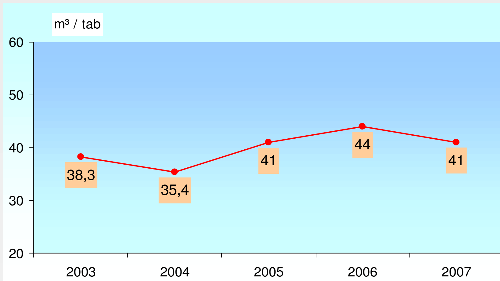
Fig. 5 - Evolução do Consumo de Gás Natural Forno Aquecimento Tarugo
