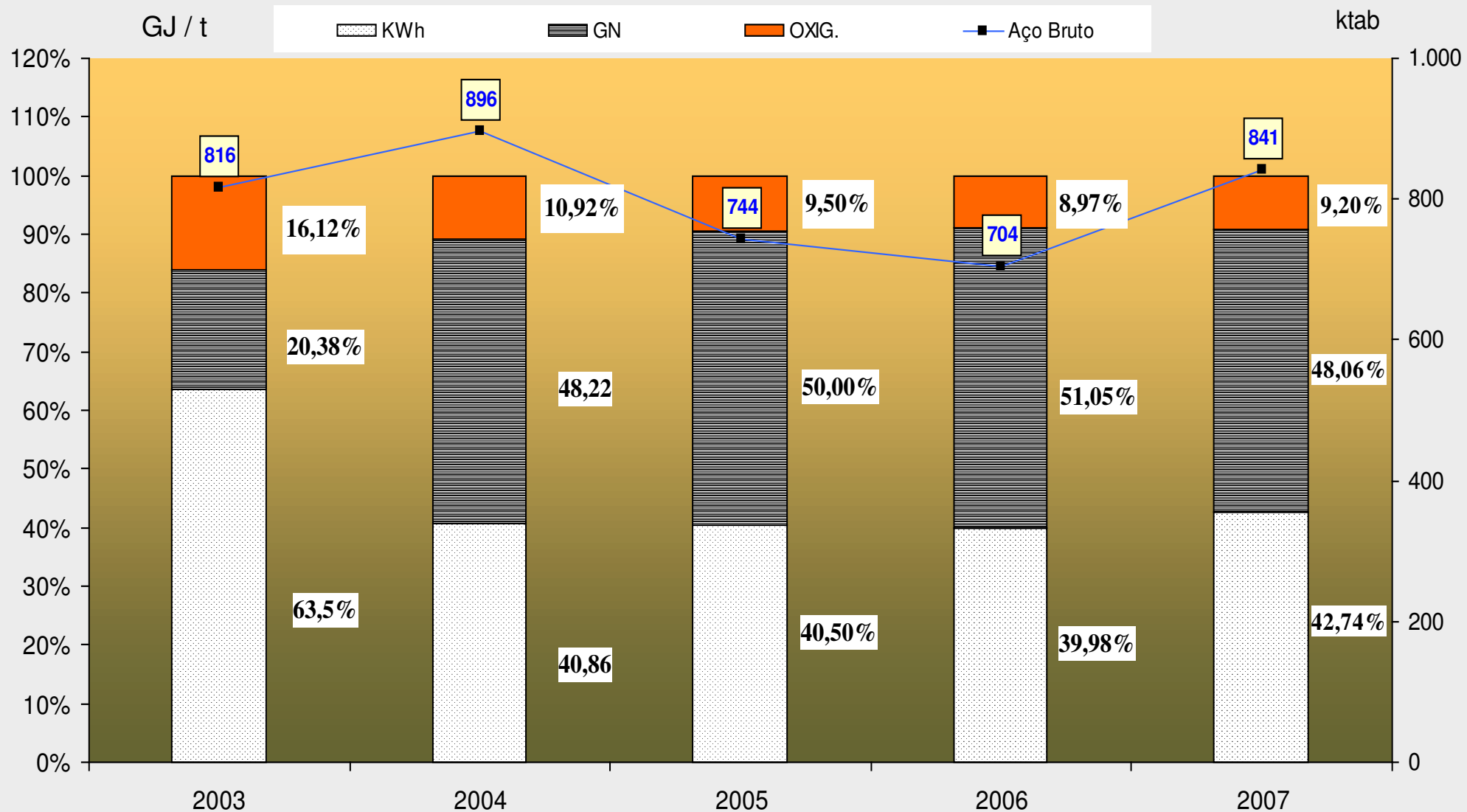
Fig. 1 - Evolução do Consumo de Energia Primária
