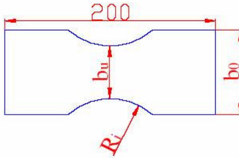
Figura 4. Modelo da geometria dos corpos de prova utilizado no ensaio de Nakazima. Unidades em mm. (5)
