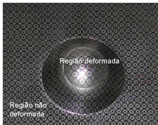
Figura 5. Corpo de prova gravado com malha circular, com regiões deformadas e não deformadas. (7)
