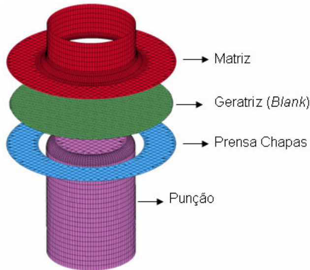
Figura 7. Esboço dos componentes da ferramenta utilizada no trabalho. (9)
