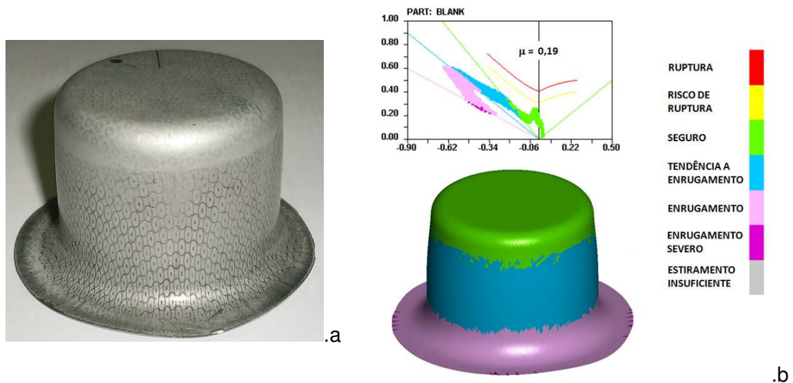
Figura 13. Copo de aço BH 180 produzida no processo sem lubrificação e da peça simulada.
