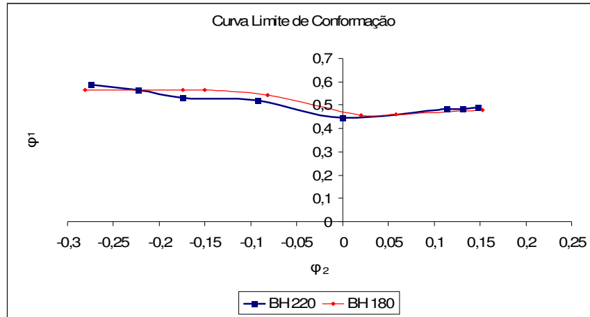
Figura 10. Sobreposição das CLC dos aços BH 180 e BH 220.
