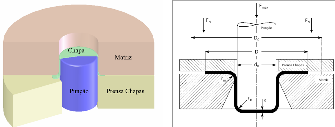
Figura 6.a. Croqui do processo de estampagem profunda utilizada para análise. b. Ilustração dos parâmetros do cálculo da força máxima. (9)
