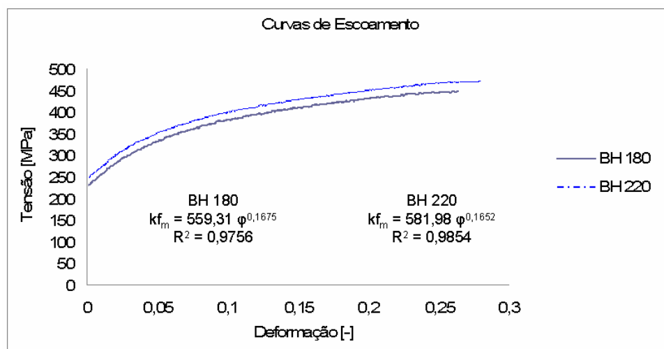
Figura 8. Curva tensão verdadeira x deformação verdadeira. Espessura 0,75mm.
