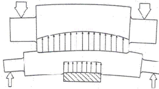
Figura 3 – Flexão dos cilindros de trabalho e encosto durante o processo de laminação. (4)
