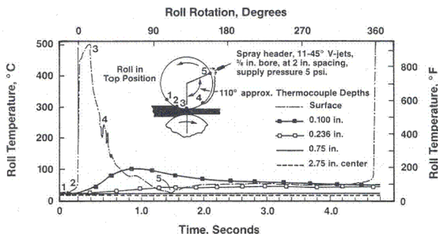
Figura 2 – Variação da temperatura do cilindro de trabalho, em diferentes posições da superfície, durante a primeira revolução. (4)
