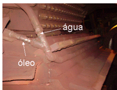
Figura 5 – Detalhe do header superior de entrada do sistema de lubrificação dos cilindros de trabalho do Steckel.
