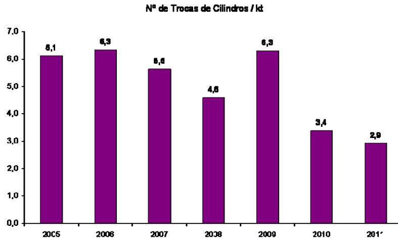
Figura 9 – Evolução do número de trocas de cilindros por mil toneladas laminadas.
