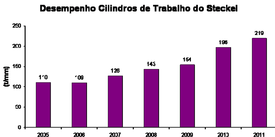
Figura 8 – Evolução do desempenho médio anual dos cilindros de trabalho do Steckel.
