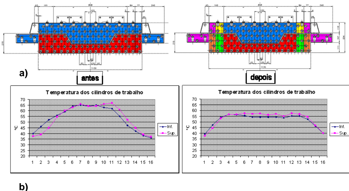
Figura 4 – a) chuveiro de refrigeração dos cilindros de trabalho (antes – 2 zonas; depois 6 zonas). b) Perfil de temperatura ao longo da mesa do cilindro de trabalho após campanha de laminação de aço inox 304, antes e após as modificações dos chuveiros.
