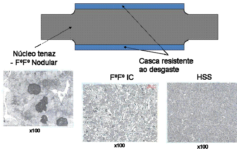
Figura 1 – Constituição básica de um cilindro de trabalho para laminação de tiras a quente. Detalhe da microestrutura do núcleo e da casca.
