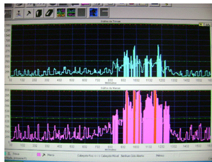
Figura 6 – Tela do Eddy Current indicando ocorrência de trincas/marcas.
