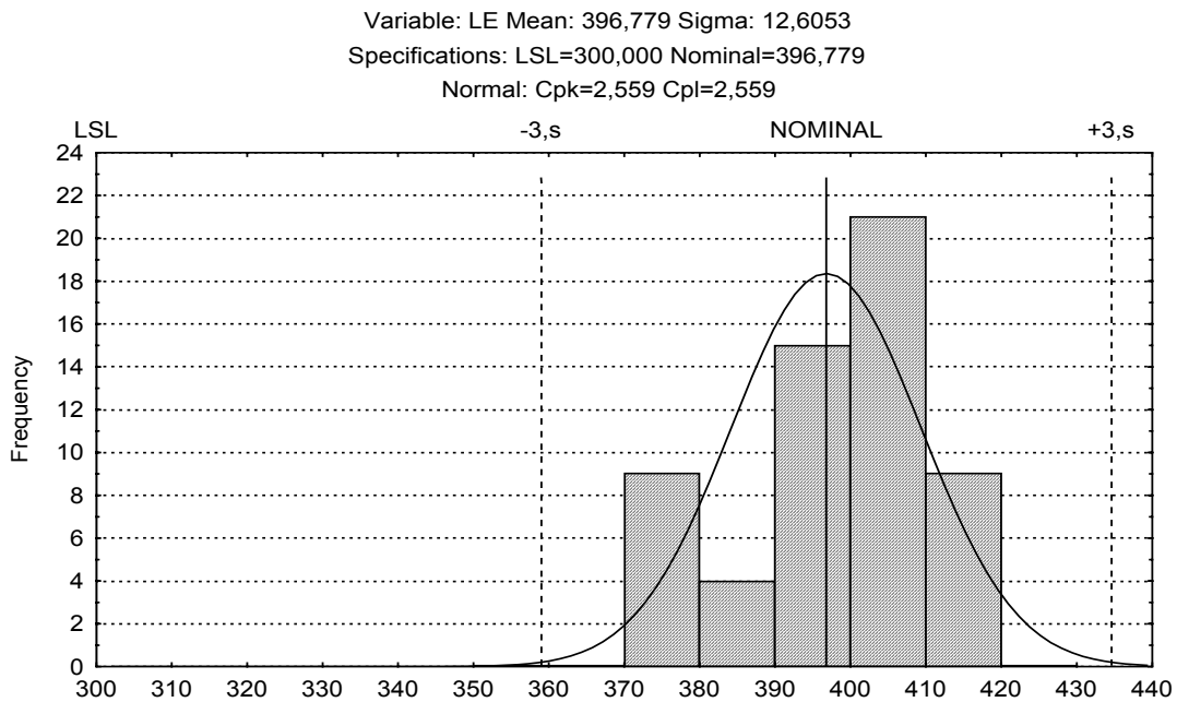
Figura 1. Distribuição de limite de escoamento obtida para o material COS-AR-COR 300. Note-se o nível de capacidade C_{pk} superior a 2,5.
