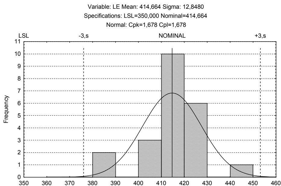
Figura 4. Distribuição de limite de escoamento obtida para o material COS-AR-COR 350. Note-se o nível de capacidade C_{pk} superior a 1,6.
