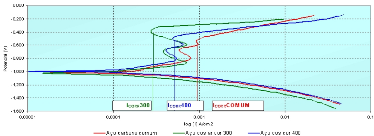
Figura 7. Curvas de polarização obtidas para amostras de aço A36, COS-AR-COR 300 e COS-AR-COR 400 imersas em solução de NaCl a 0,1M.
