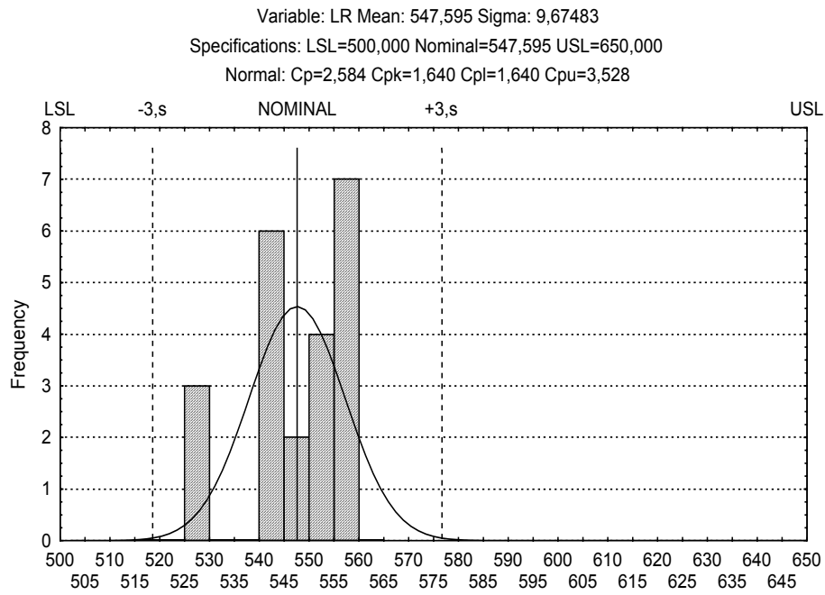
Figura 5. Distribuição de limite de resistência obtida para o material COS-AR-COR 350. Note-se o nível de capacidade C_{pk} superior a 2,5.
