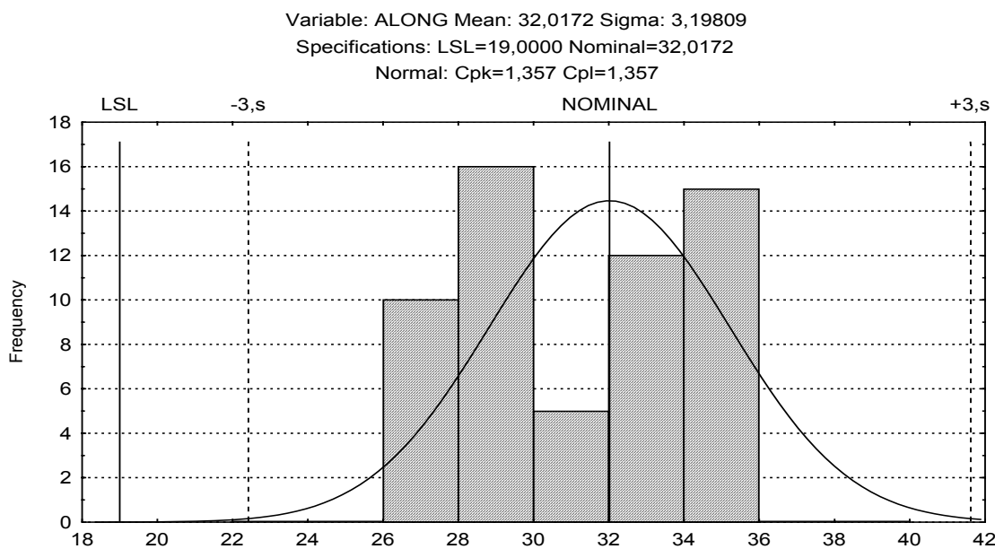
Figura 3. Distribuição de alongamento total obtida para o material COS-AR-COR 300. Note-se o nível de capacidade C_{pk} superior a 1,3.
