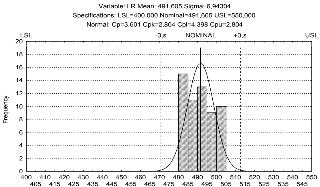
Figura 2. Distribuição de limite de resistência obtida para o material COS-AR-COR 300. Note-se o nível de capacidade C_{pk} superior a 2,8.
