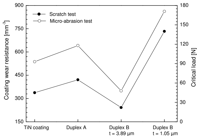
Figura 4. Comparação entre a carga crítica de riscamento e a resistência ao desgaste microabrasivo
