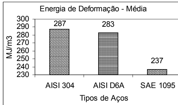
Figura 5. Energia de deformação média na etapa de desbaste dos aços AISI 304, AISI D6A e SAE 1095, entre os dias 01/01/05 a 30/06/05, em 7 passes e esboço de 28 mm.
