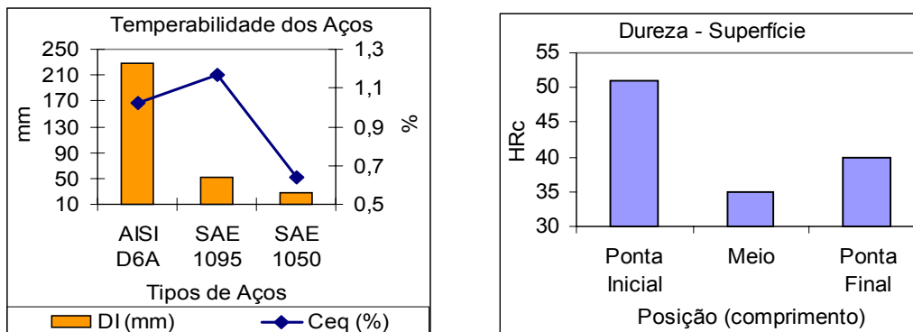
Figura 6. A esquerda, comparação da temperabilidade (DI em mm) e carbono equivalente (Ceq em %) dos aços AISI D6A, SAE 1095 e SAE 1050. A direita, evolução da dureza típica ao longo do comprimento das bobinas de AISI D6A.
