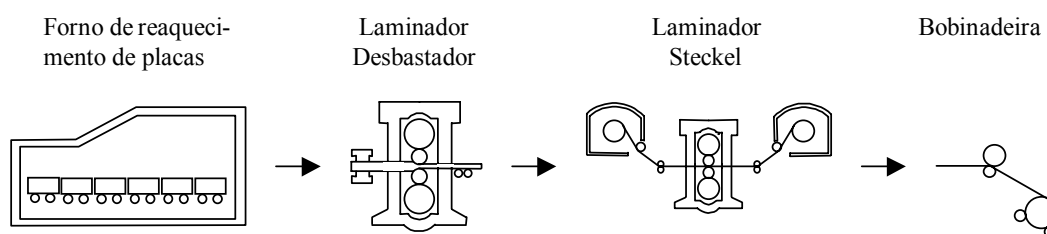
Figura 2. Fluxograma simplificado do processo de laminação a quente.
