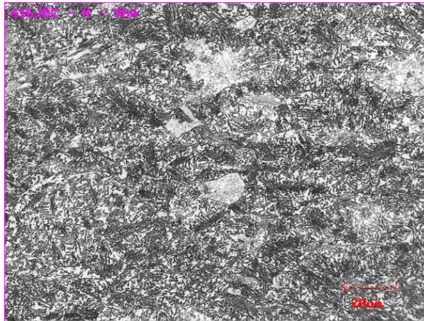
Figura 7. Microestrutura típica do centro das bobinas de D6A.
