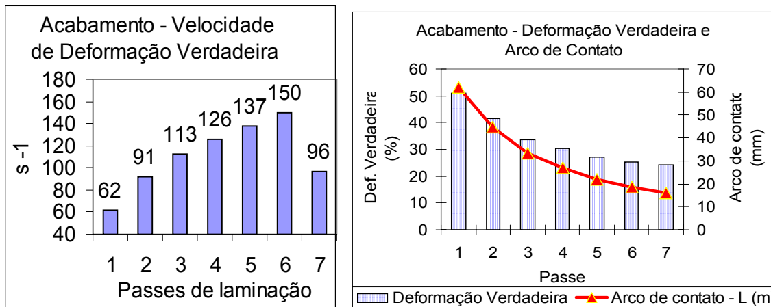
Figura 4. Velocidade de deformação verdadeira, deformação verdadeira e arco de contato na laminação de acabamento de aço AISI D6A, com espessura inicial de 28 mm (esboço) e final de 2,65 mm (bobina a quente).
