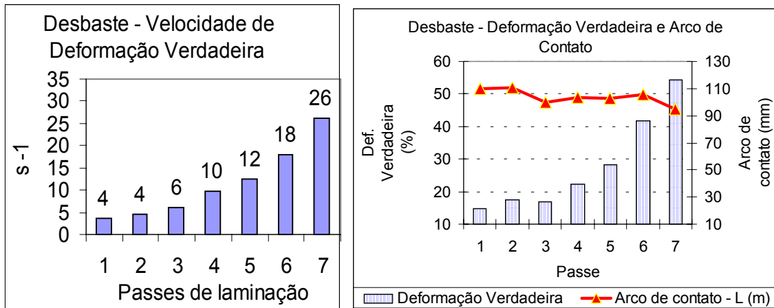
Figura 3. Velocidade de deformação verdadeira, deformação verdadeira e arco de contato na laminação de desbaste de aço AISI D6A, com espessura inicial de 200 mm (placa) e final de 28 mm (esboço).
