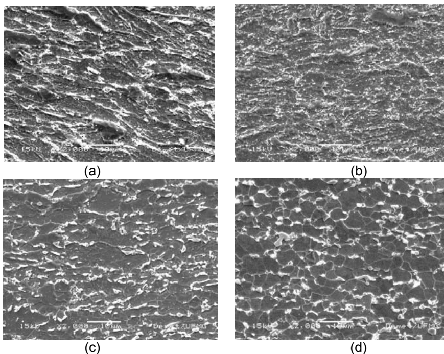
Figura 3. Micrografias obtidas no MEV e atacada com nital 2%. Amostras do metal base recozidas a 550°C por 5 min (a), 550°C por 3 h (b), 800°C por 5 min (c) e 800°C por 3 h (d).
