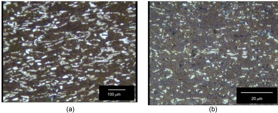
Figura 10. Micrografias ópticas. Ataque com reativo de LePera de amostras na ZTA recozidas a 550°C e 800°C durante 5 min com velocidades de soldagem iguais a 40 e 20 cm/min, respectivamente.
