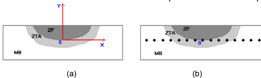
Figura 2. (a) Eixos utilizados para o levantamento do perfil microdureza ao longo da ZTA. (b) Exemplo de disposição das impressões. ZF – zona fundida; ZTA – zona termicamente afetada; MB – metal de base.
