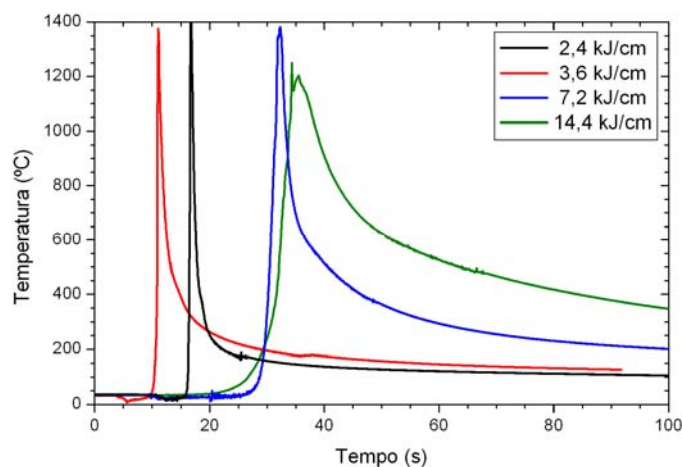
Figura 5. Exemplos de ciclos térmicos medidos durante os testes de soldagem.
