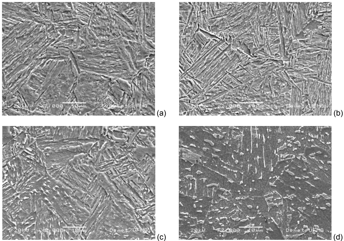
Figura 7. Microestrutura da CGZTA (MEV - seção transversal). Energias de soldagem: (a) 2,4; (b) 3,6; (c) 7,2 e (d) 14,4 kJ/cm. Ataque: Nital 2%. Aumento: 2000x. Metal base: 550°C/3h.
