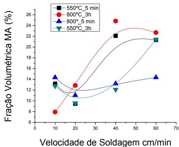
Figura 9. Fração Volumétrica de constituinte MA na ZTA para as diferentes condições de recozimento e velocidade de soldagem.
