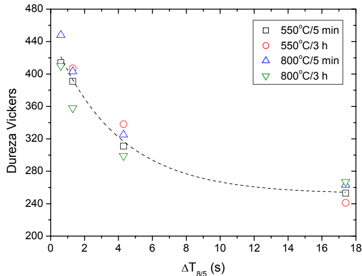
Figura 12. Variação de dureza máxima da ZTA dos aços submetidos aos diferentes tratamentos em função do tempo de resfriamento durante a soldagem entre 800 e 500°C.
