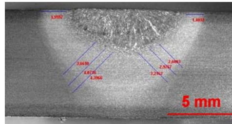
Figura 6. Seção transversal da solda em um corpo de prova soldado com energia de 7,2 kJ/cm.
