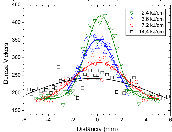
Figura 11. Variação de dureza nas ZTA's do aço recozido a 800°C durante 3 h.
