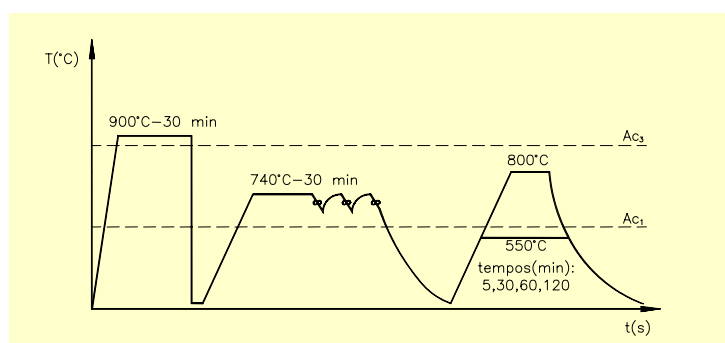
Figura 1. Esquema de processamento térmico e mecânico aplicado ao material investigado.
