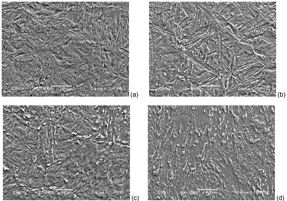
Figura 8. Microestrutura da CGZTA (MEV - seção transversal). Energias de soldagem: (a) 2,4; (b) 3,6; (c) 7,2 e (d) 14,4 kJ/cm. Ataque: Nital 2%. Aumento: 500x. Metal base: 800°C/3h.
