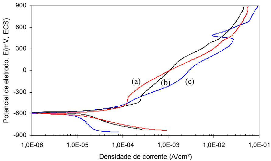
Figura 2 - Curvas de polarização potenciodinâmica; sistemas: aços AISI 321 (a) 316L (b); 304L (c)/água amoniacal; 0,17mV/s; temperatura ambiente.
