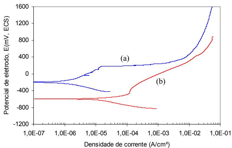
Figura 4 - Curvas de polarização potenciodinâmica; sistemas: aço AISI 321/soluções aquosas com 3,5% (peso) de NaCl (a) e água amoniacal (b); 0,17mV/s; temperatura ambiente.
