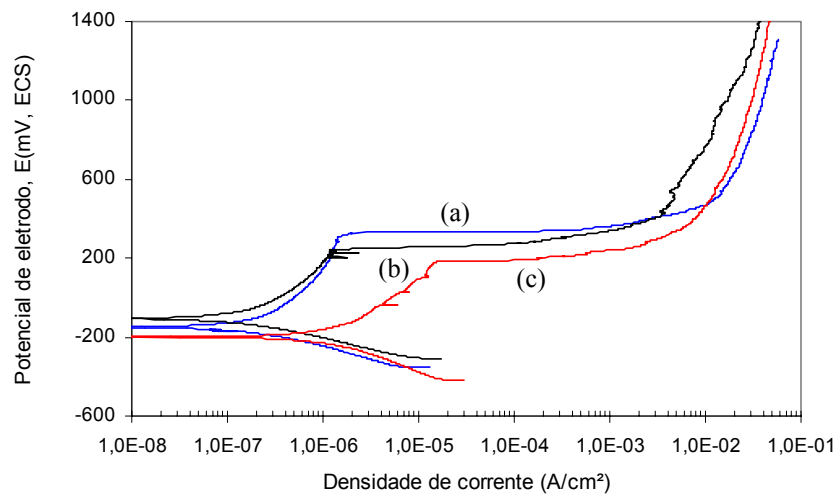
Figura 3 - Curvas de polarização potenciodinâmica; sistemas: aços AISI 304L (a); 316L (b); 321 (c)/soluções aquosas com 3,5% (peso) de NaCl; 0,17mV/s; temperatura ambiente.
