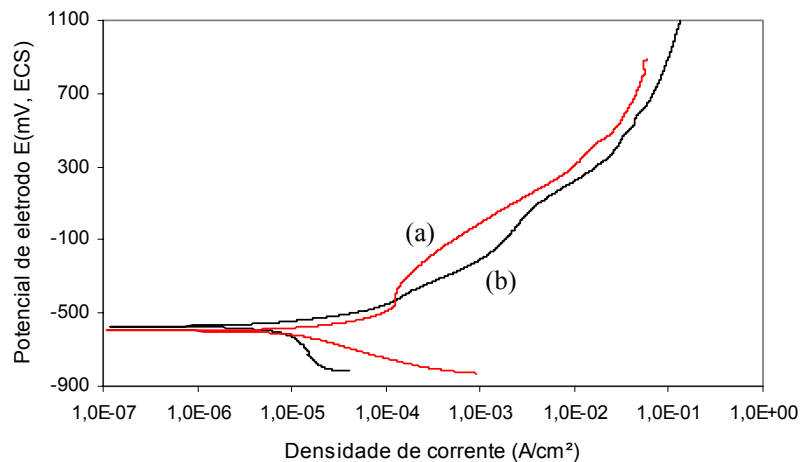
Figura 5 - Curvas de polarização potenciodinâmica; sistemas: (a) aço no estado de entrega do tipo AISI 321 e (b) o de uma tubulação da coqueria (Tubo 4) / água amoniacal; 0,17mV/s; temperatura ambiente.
