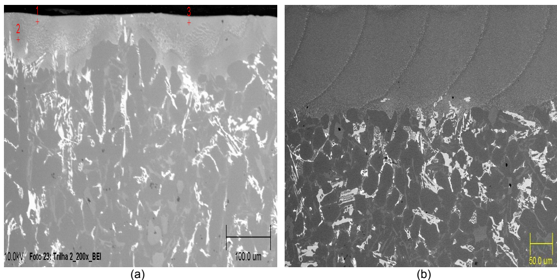
Figura 4. Micrografias da seção transversal da liga Al-Si obtida por MEV (elétrons retroespalhados) (a) sob a condição TRL2; e (b) sob a condição TRL4.
