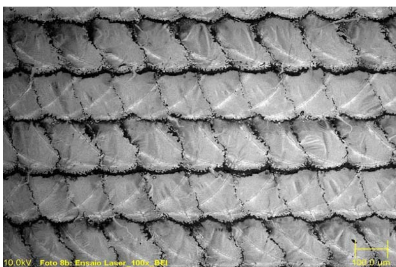
Figura 3. Micrografia eletrônica de varredura (elétrons retroespalhados) da seção longitudinal da amostra irradiada com trilhas (condição TRL4).
