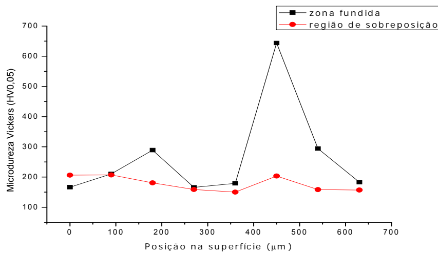
(c) Condição TRL4
