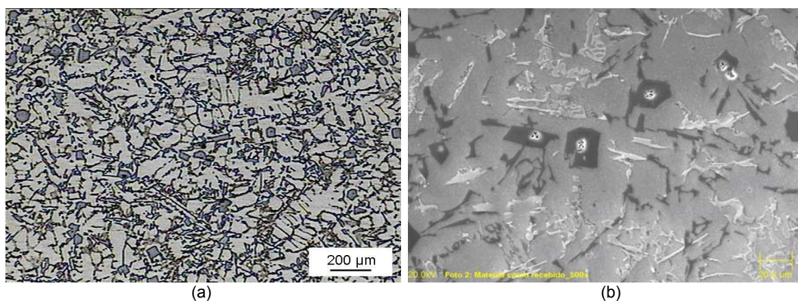
Figura 2. Microestrutura da liga Al-Si no estado de como recebida com ataque químico (HF5%) obtida por MO e MEV/ elétrons secundários, respectivamente.
