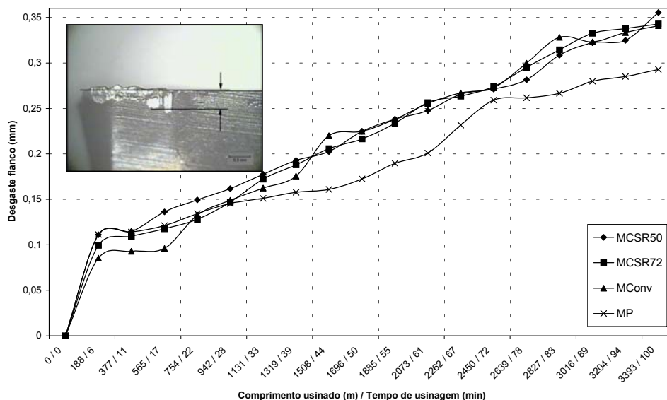
Figura 8. Curvas de desgaste para velocidade de corte de 34 m/min (valores médios referente a 1ª e 2ª baterias de testes) [4].
