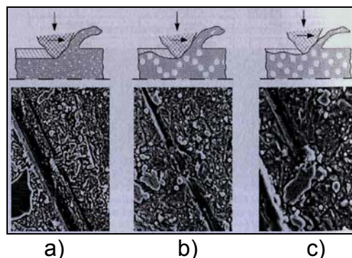
Figura 7. Influência do tamanho e distribuição dos carbonetos na resistência ao desgaste dos aços ferramenta. a) Carbonetos muito finos; b) Carbonetos grosseiros orientados com formação em rede; c) Carbonetos grosseiros homogeneamente distribuídos [24,25].
