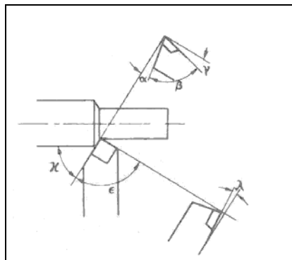
Figura 2. Representação simplificada da geometria das ferramentas (pastilha + suporte) utilizadas nos experimentos [4].
