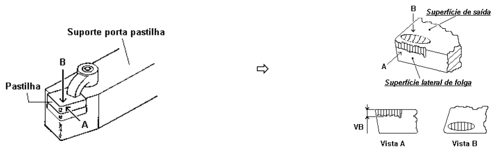
Figura 3. Esquema ilustrativo dos locais de desgaste na pastilha. A (vista A) - Desgaste de flanco (superfície lateral de folga); B (vista B) - Desgaste de cratera (superfície de saída) [4] .
