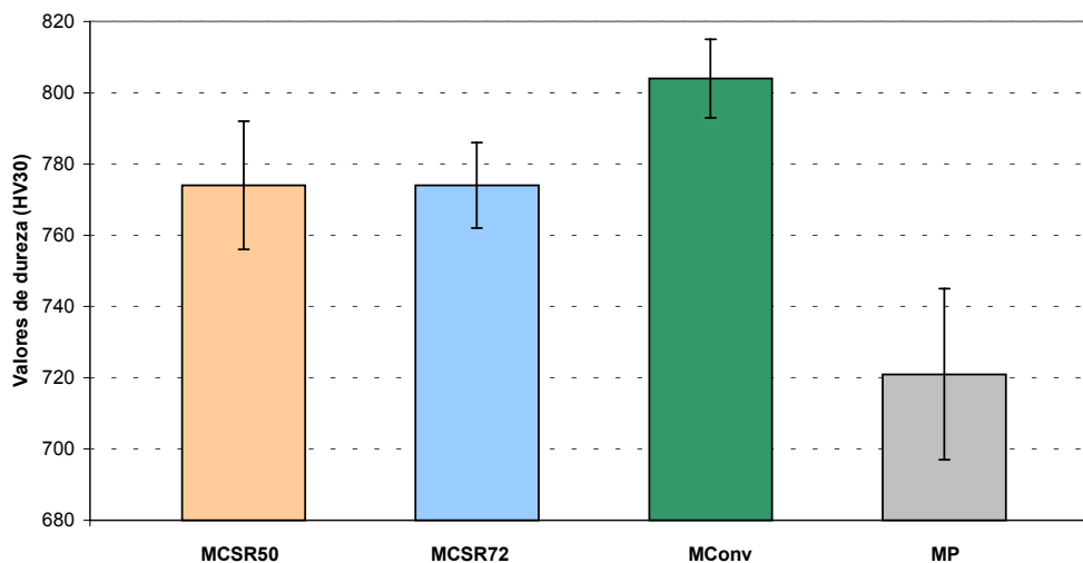
Figura 4. Dureza dos materiais após tratamento térmico (têmpera e revenimento) [4] .
