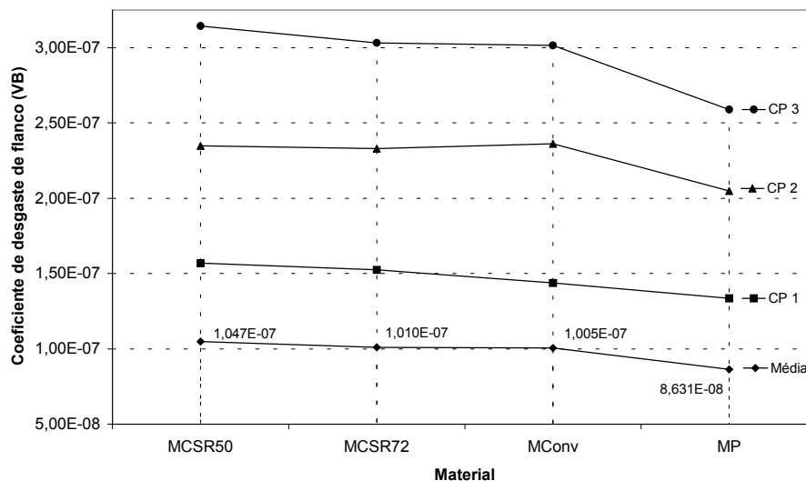
Figura 9. Valores de “coeficiente de desgaste” relativos aos testes com velocidade de corte de 34 m/min (dados cumulativos) [4] .
