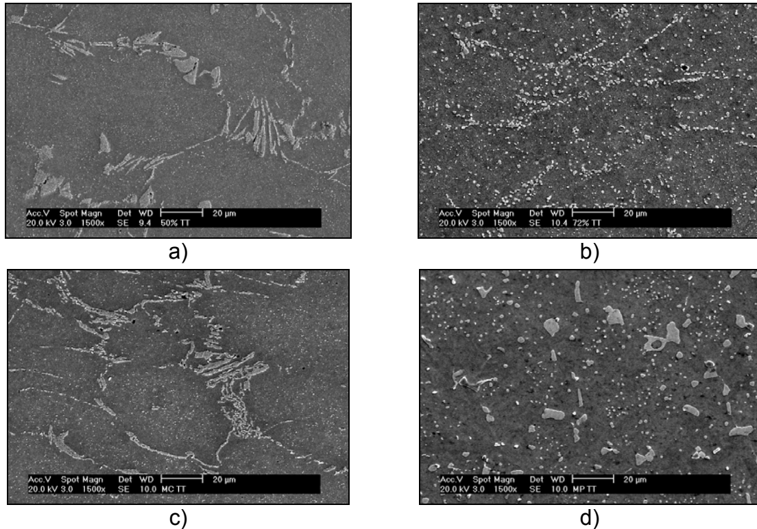
Figura 6. Micrografia eletrônica de varredura do material após tratamento térmico de têmpera e revenimento – sem ataque. a) MCSR50. b) MCSR72. c) MConv. d) MP.
