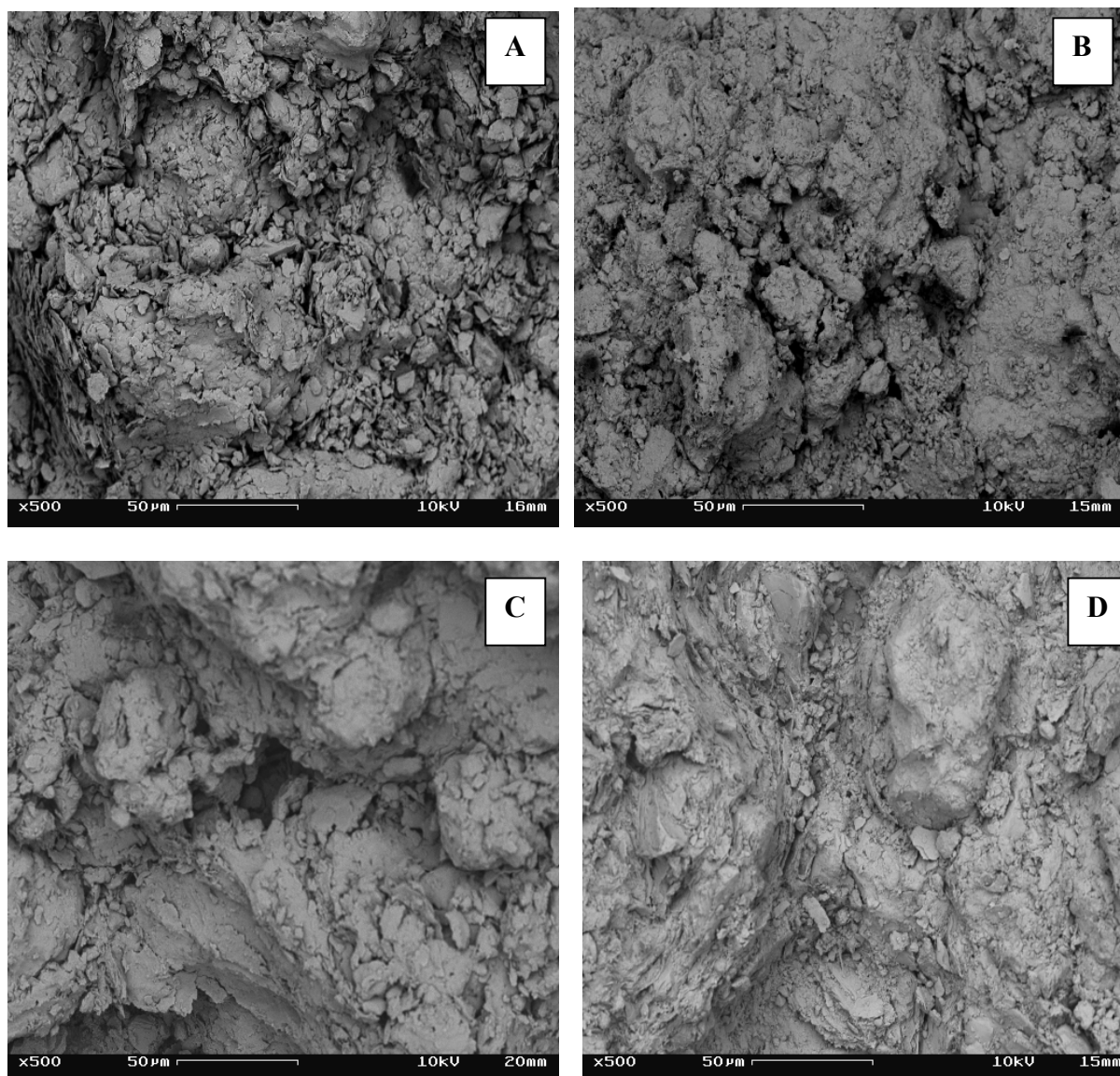
Figura 2: Micrografias obtidas por MEV da região de fratura das cerâmicas. (a) Portugal; (b) Santa Catarina; (c) Piauí; (d) Campos.
