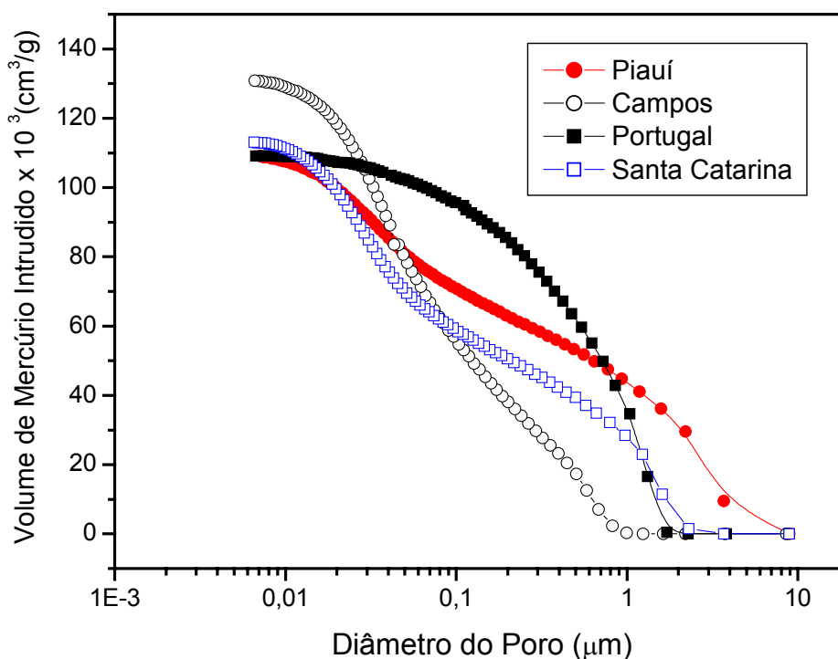
Figura 4: Curvas de porosimetria de mercúrio das cerâmicas queimadas a 975°C.
