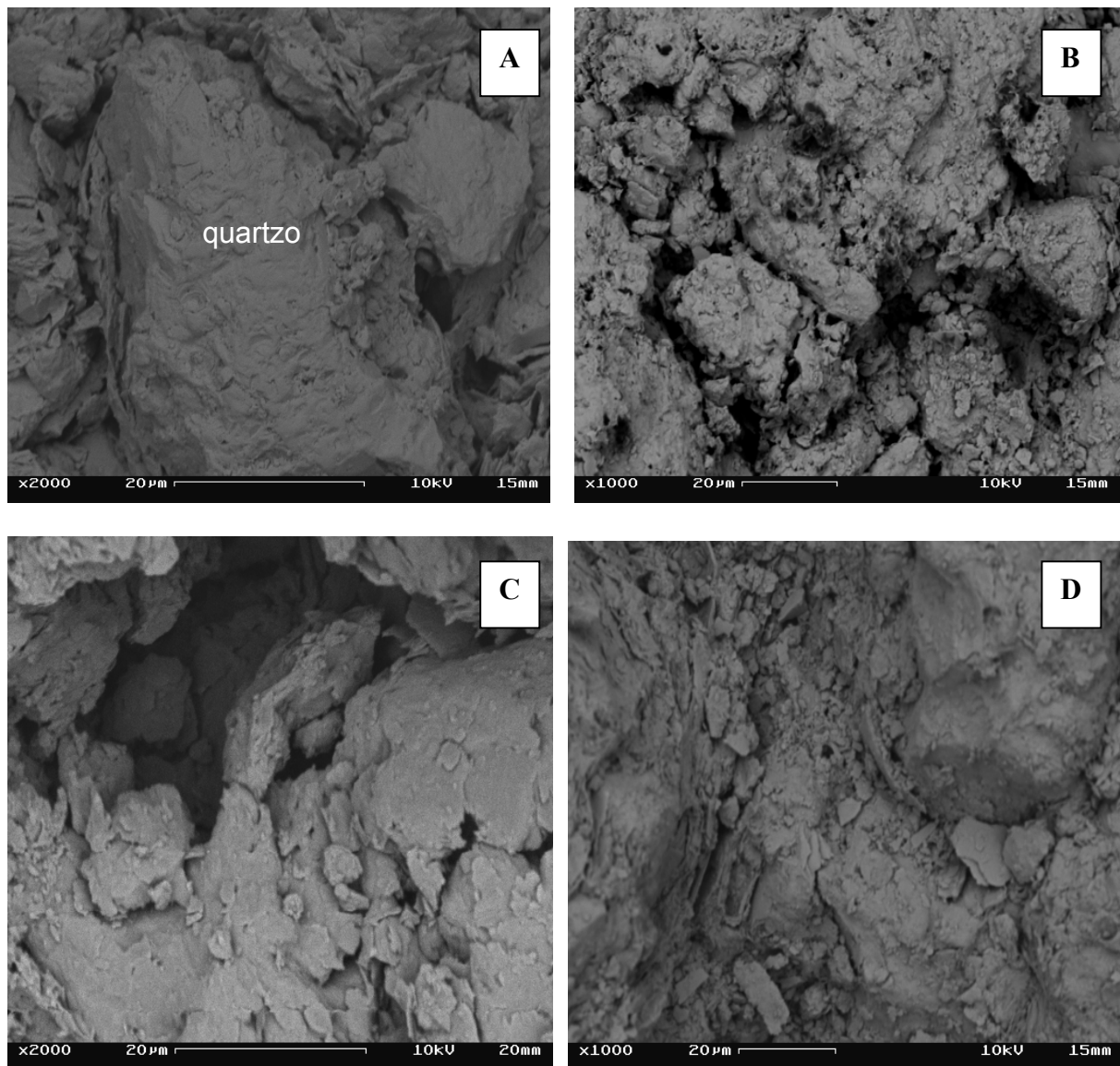
Figura 3: Micrografias obtidas por MEV das massas cerâmicas. (a) Portugal; (b) Santa Catarina; (c) Piauí; (d) Campos.
