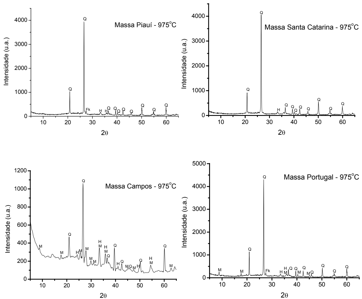
Figura 1: Difratograma de raios-X das massas cerâmicas queimadas a 975°C.
