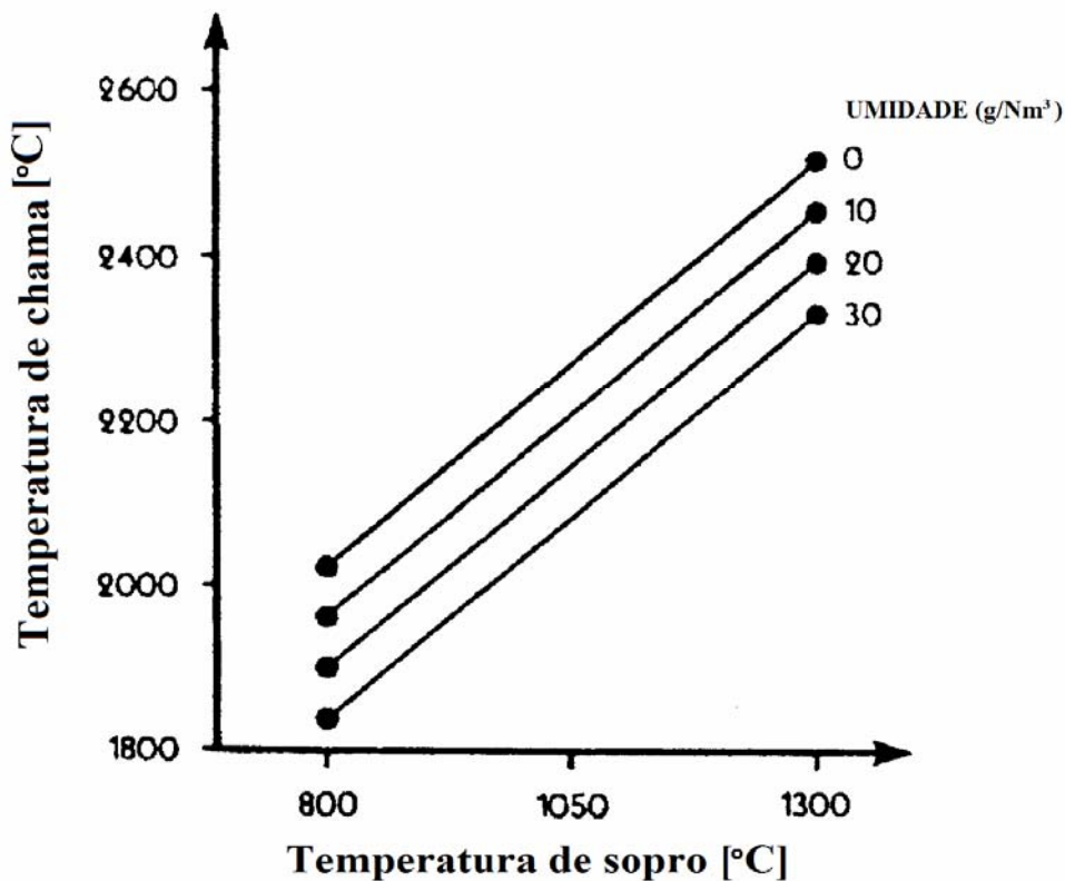
Figura 1 Relação da temperatura de chama com a temperatura de sopro. (1)
