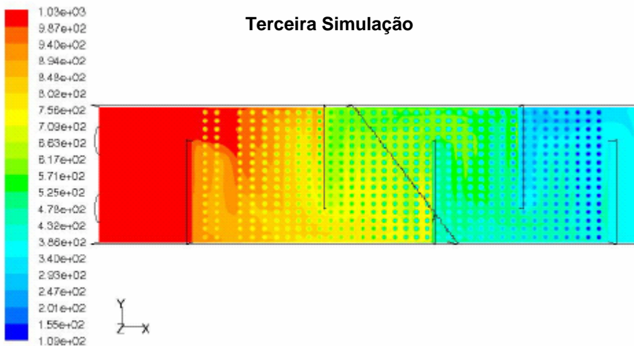
Figura 6 Evolução do perfil de temperatura ao longo do Glendon – Vista de planta
