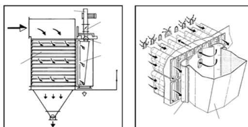
Figura 5. Sistema de limpeza móvel utilizando soprador.
