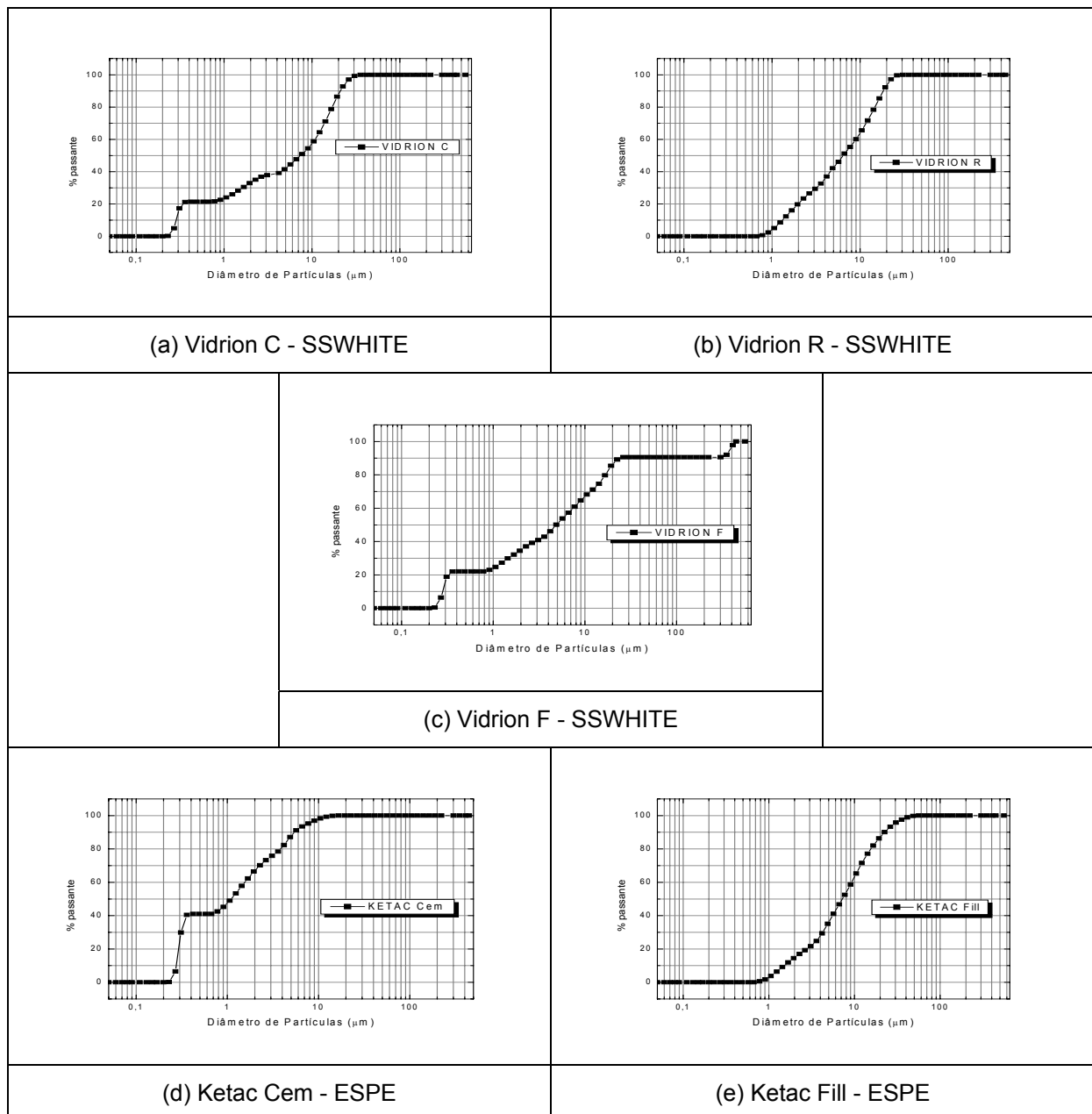
Figura 3. Curvas de % passante versus diâmetro de partículas dos cimentos
