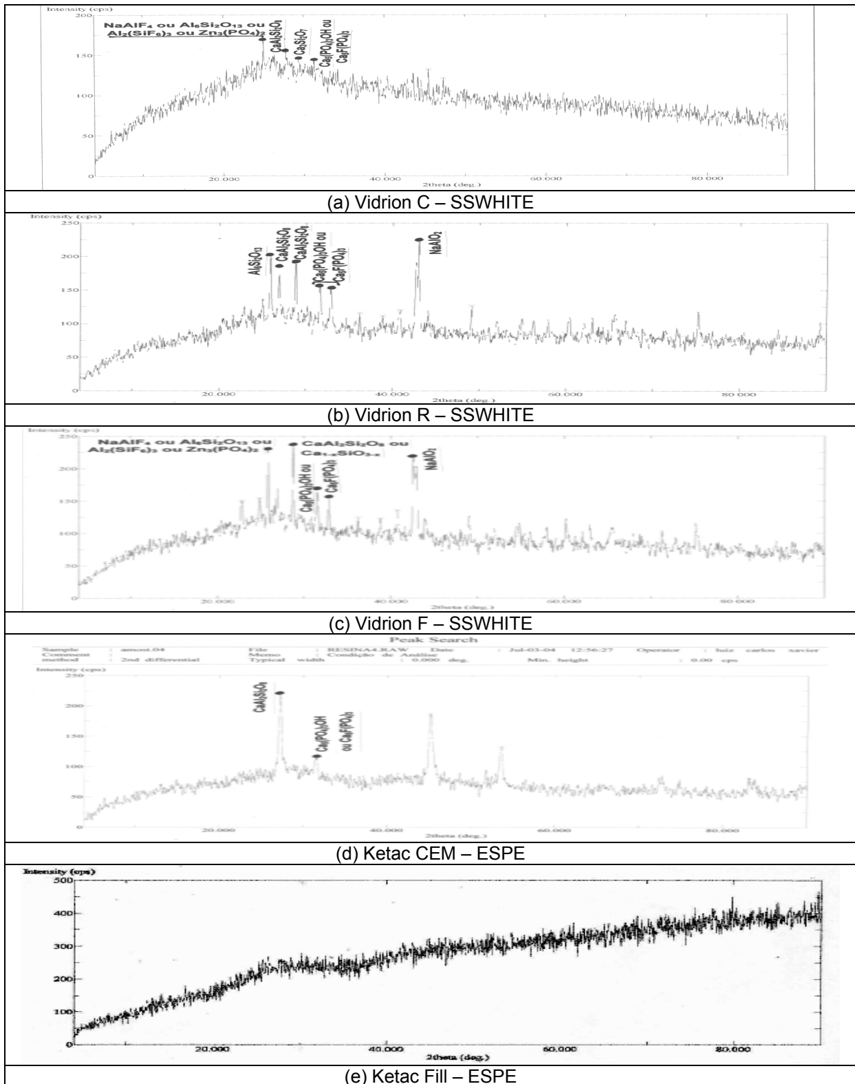
Figura 2. Difratomogramas de raios-X dos pós dos cimentos de ionômero de vidro.
