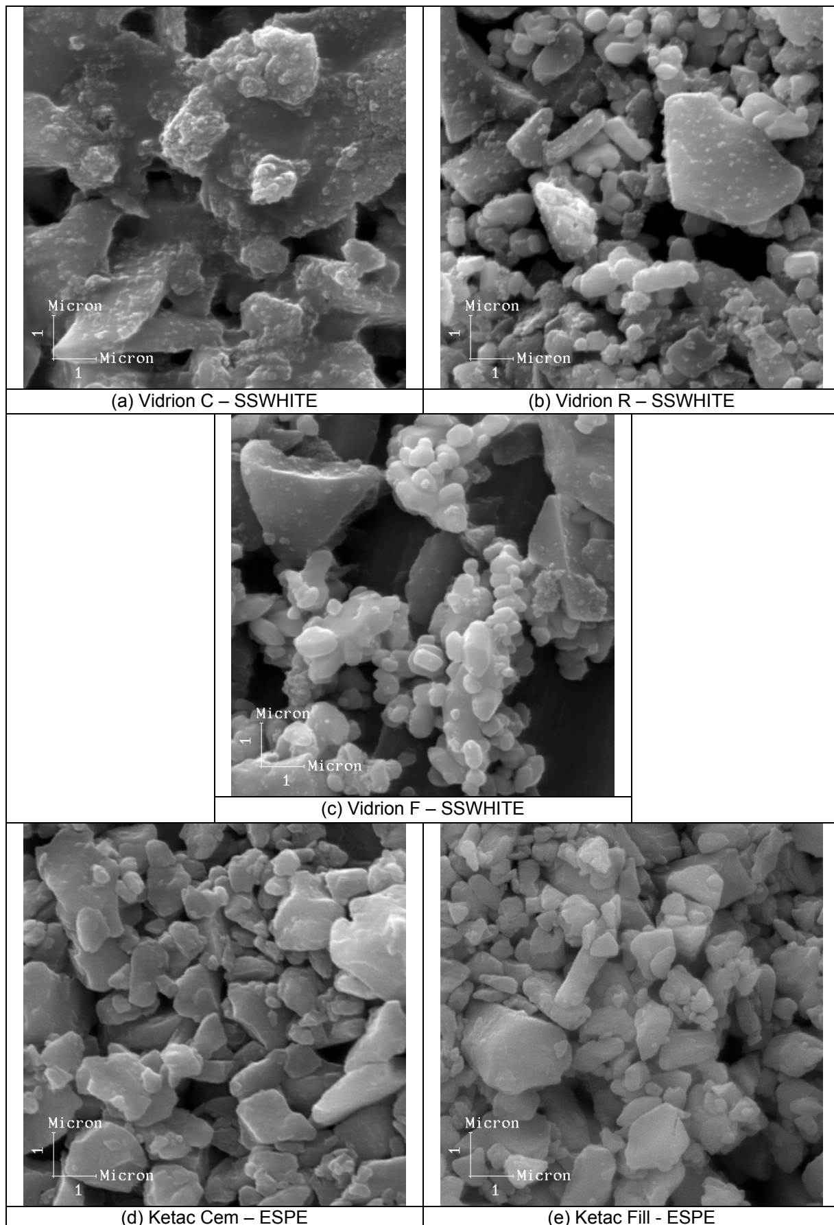
Figura 1. Micrografia MEV dos pós dos cimentos de ionômeros de vidro.
