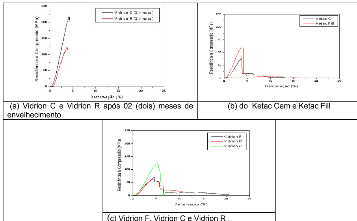
Figura 4. Curvas de resistência à compressão versus deformação dos cimentos.
