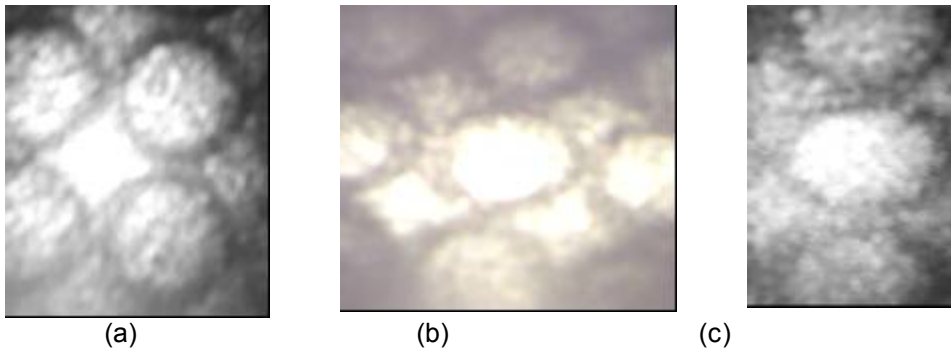
Figura 17. Círculos gravados por corrosão eletroquímica observados em diversas regiões da peça estampada: (a) base; (b) curvatura entre lateral e fundo; (c) lateral
