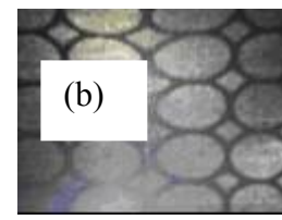
Figura 16. Amostras de tração deformadas plasticamente, observadas em projetor de perfil (10X): (a) corrosão eletroquímica; (b) serigrafia; (c) roto-gravura
