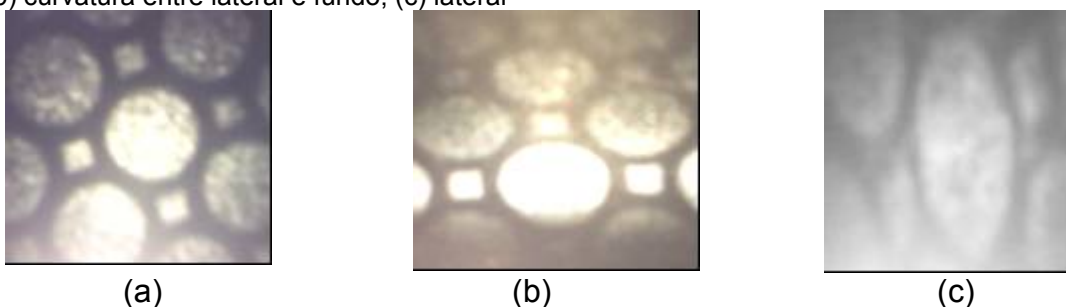
Figura 19. Círculos gravados por roto-gravura observados em diversas regiões da peça estampada: (a) base; (b) curvatura entre lateral e fundo; (c) lateral
