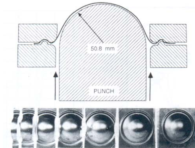
Figura 3. Geometrias de corpos de prova submetidos a ensaio de estiramento [8]
