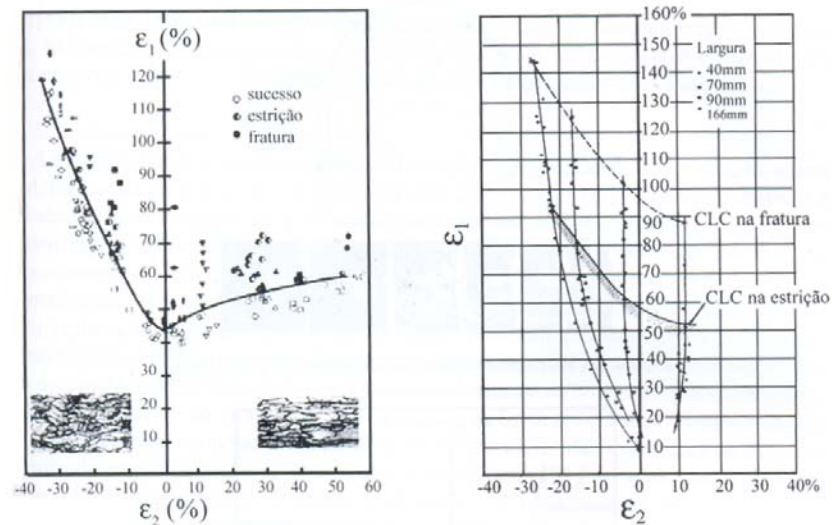
Figura 1. CLC para aço Carbono. [3] Figura 2. Caminho de deformação [7]
