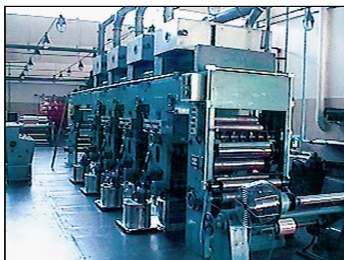
Figura 7. Equipamento gráfico para roto-gravura. (10)
