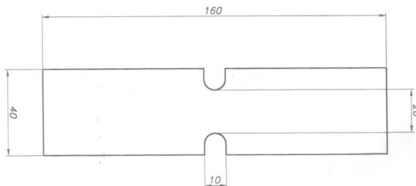
Figura 4. Geometria e dimensões das amostras para ensaios de tração.
