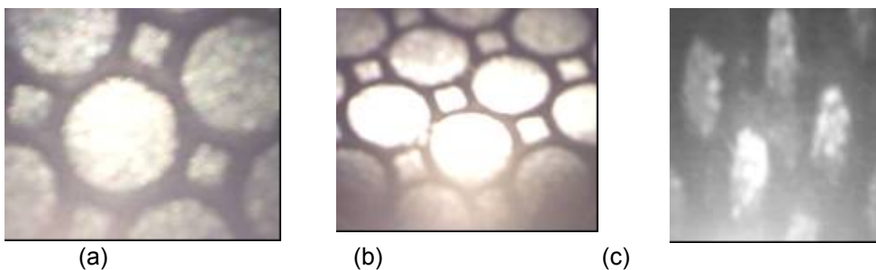
Figura 18. Círculos gravados por serigrafia observados em diversas regiões da peça estampada: (a) base; (b) curvatura entre lateral e fundo; (c) lateral
