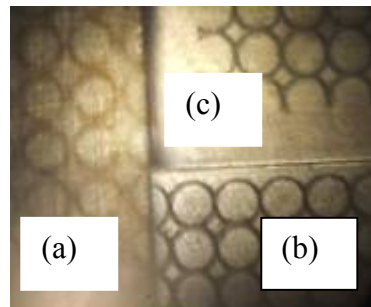
Figura 15. Amostras de tração isentas de deformação plástica observadas em projetor de perfil (10X): (a) corrosão eletroquímica; (b) serigrafia; (c) roto-gravura.
