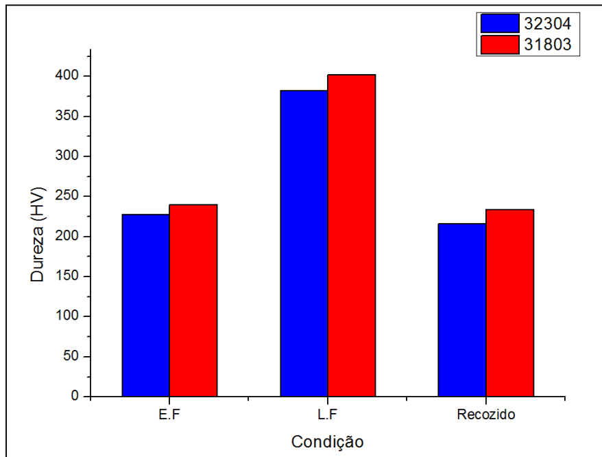
Figura 4. Ensaio de dureza.
