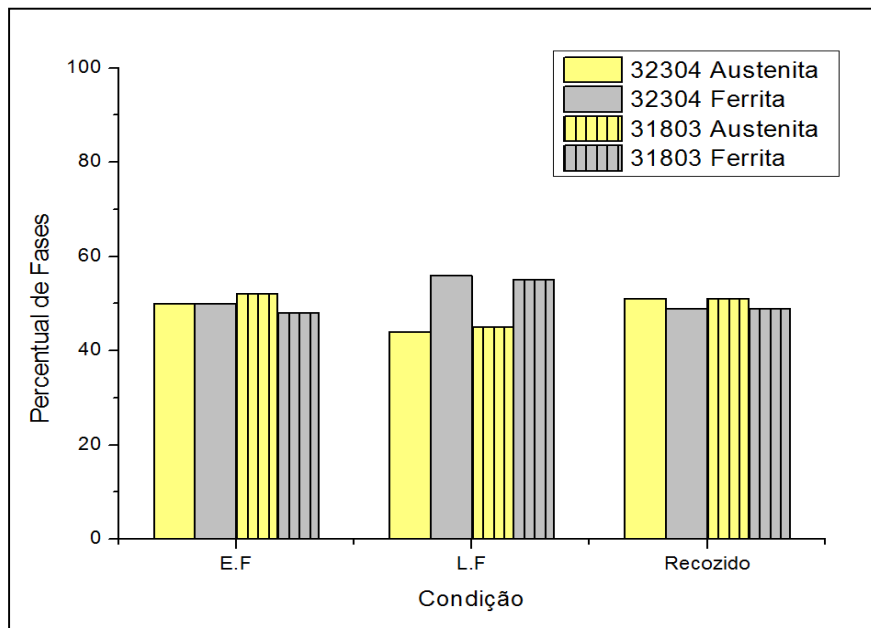
Figura 3. Fração volumétrica das fases.
