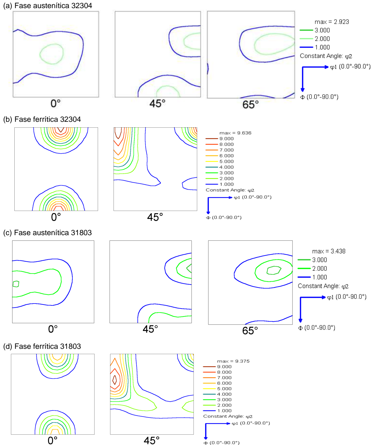
Figura 6. ODF das amostras recozidas.
