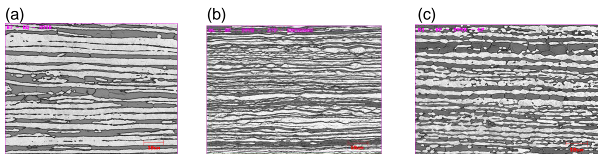
Figura 2. Aço inoxidável duplex S31803: (a) estado de fornecimento; (b) deformada (64%) e (c) recozida.
