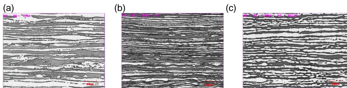
Figura 1. Aço inoxidável duplex S32304: (a) estado de fornecimento; (b) deformada (62%) e (c) recozida.
