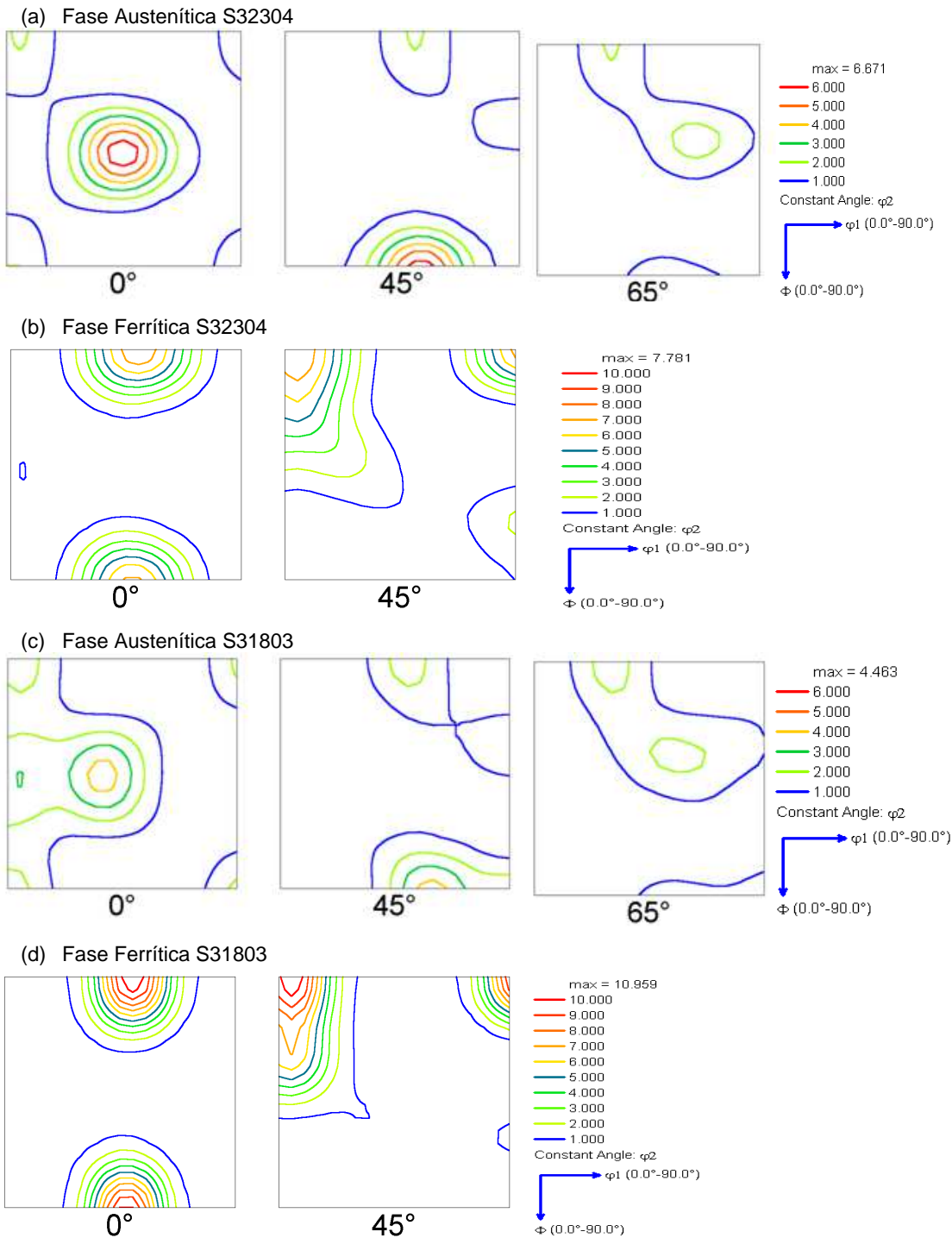
Figura 5. ODF das amostras no estado de fornecimento
