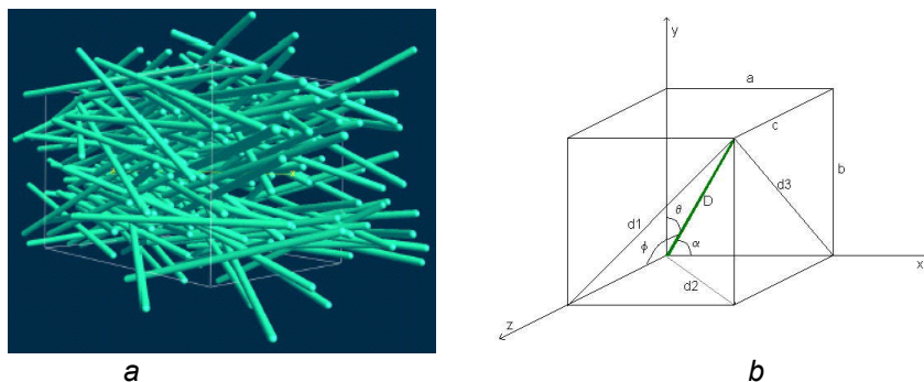
Figura 1. (a) Distribuição das fibras no compósito. (b) Fibra que representa a posição média das fibras no compósito. Casaril. (6)
