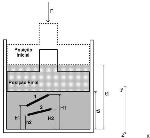
Figura 2. Alinhamento preferencial devido à compactação. Casaril. (6)
