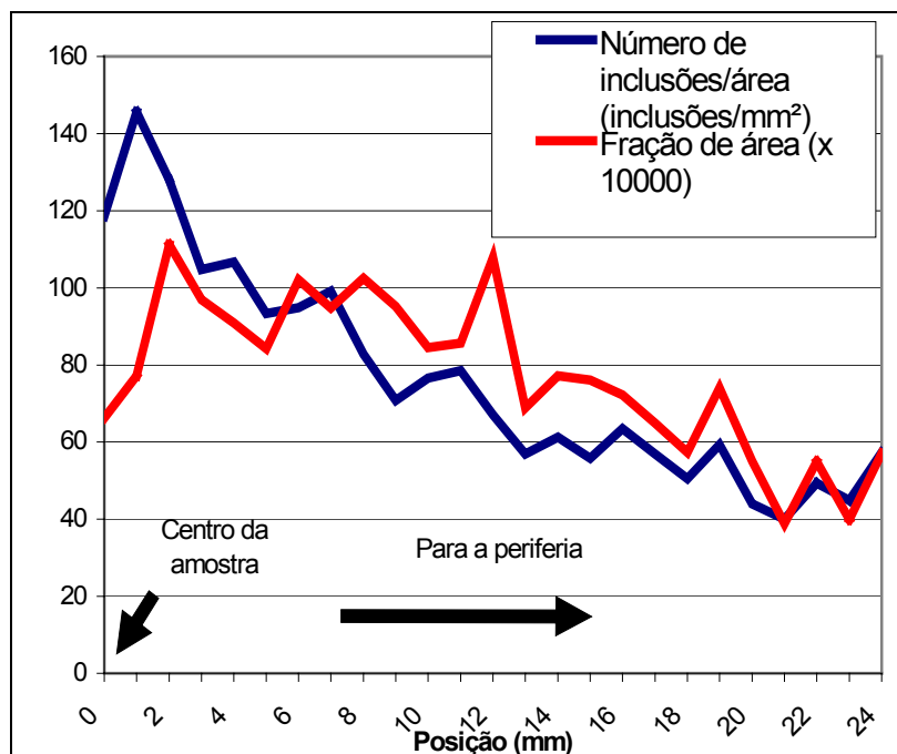
Figura 1: Evolução do número de inclusões e fração de área em função da posição, para o aço A.
