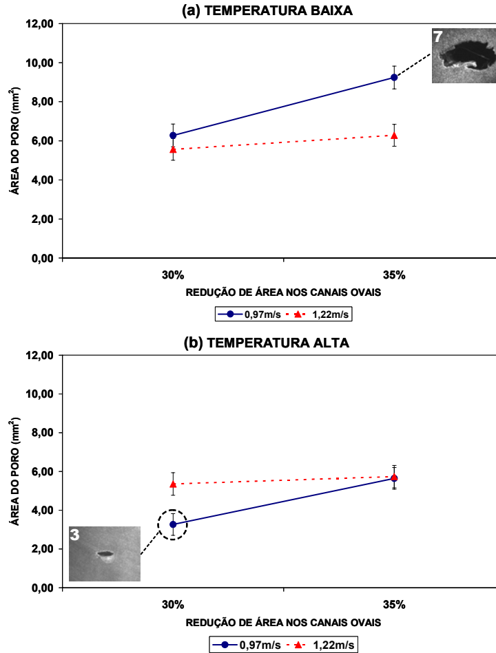
Figura 4: Diagramas de respostas da área do poro para as variáveis em seus dois níveis. (a) Temperatura baixa, e (b) Temperatura alta. O círculo tracejado indica a escolha do melhor nível para a menor área do poro remanescente para laminação em canais (fio-máquina). As linhas verticais em cada ponto representam o intervalo de confiança a 95%.
