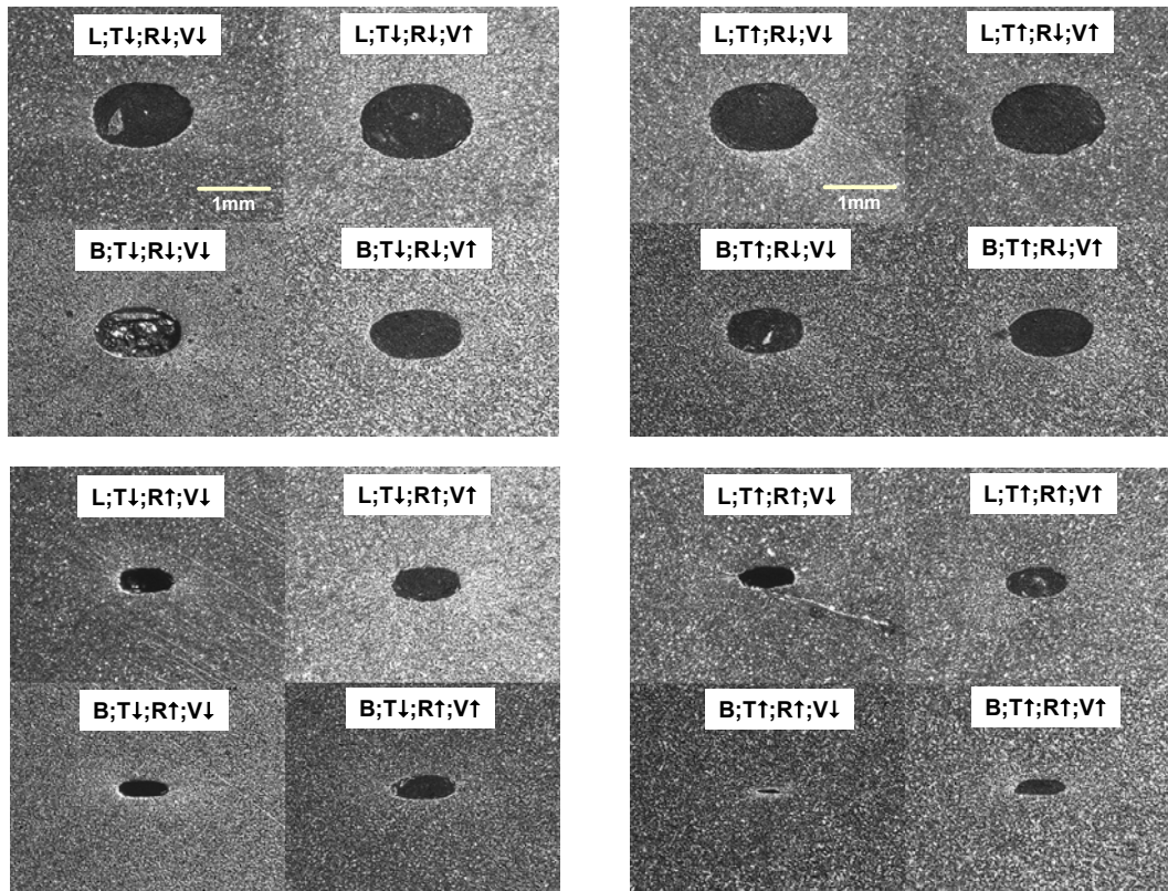
Figura 1: Microestrutura da seção transversal dos corpos de prova da laminação de planos conforme definido na Tabela 2. Ataque Nital 2%. Legenda: B: aço baixo carbono; L: aço ligado; T: temperatura; R: redução; V: velocidade. As setas indicam o nível da variável em cada ensaio (↑: alto; ↓: baixo).
