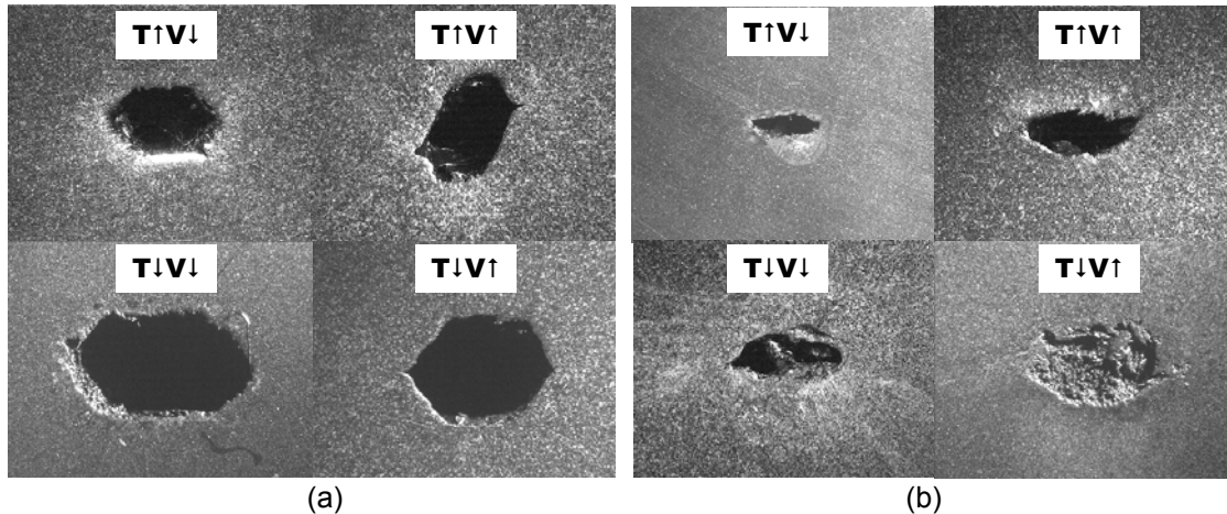
Figura 3: Microestrutura da seção transversal das amostras da laminação em canais conforme condição do ensaio da Tabela 3. Ataque: Nital 2%. (a) Redução de 35% nos canais ovais; (b) Redução de 30% nos canais ovais. Legenda: T: temperatura; V: velocidade. As setas indicam o nível de cada variável (↑: alto; ↓: baixo).
