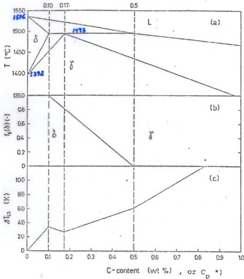
Figura 4. Diagrama Fe-C. (1)
