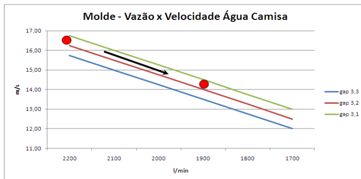
Figura 7. Vazão x velocidade de água da camisa.
