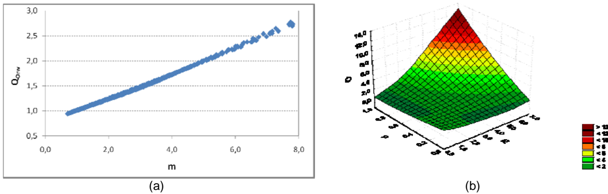
Figura 2. a) Relação Q_{ORW} x m determinada a partir dos valores de carga de laminação calculados pelo modelo de Orowan assumindo atrito de agarramento; b) Relação Q_{ORW}^{\mu} x m x \mu determinada a partir dos valores de carga de laminação calculados pelo modelo de Orowan assumindo atrito misto.
