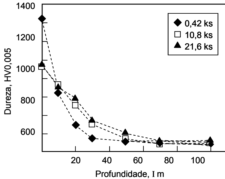
Figura 7. Perfil de endurecimento do aço AISI D2 após nitretação sob plasma.
