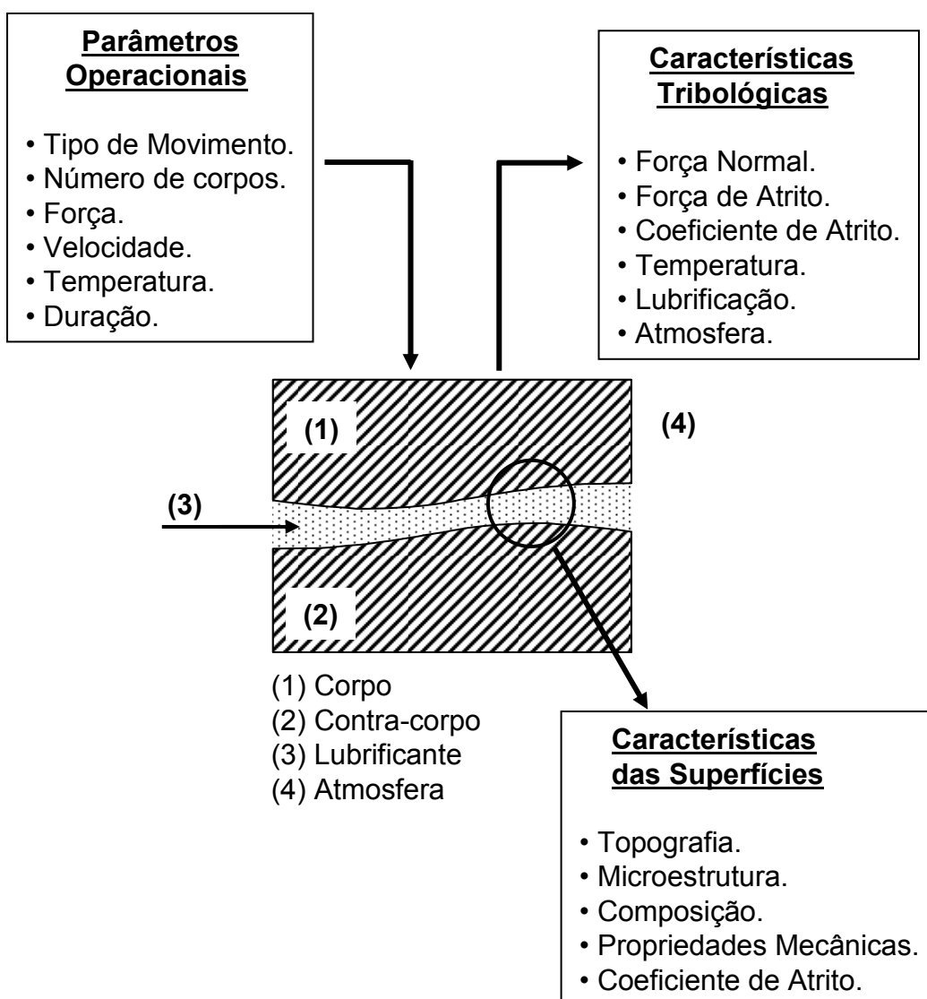
Figura 2. Principais características de um sistema tribológico.
