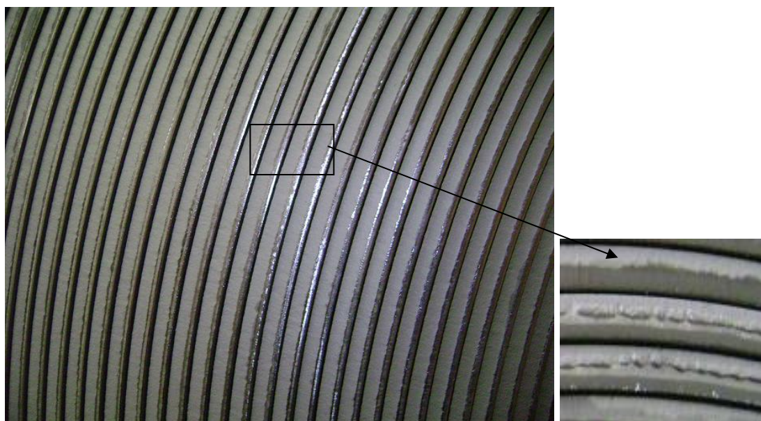
Figura 5 – Corte encaroçado.
