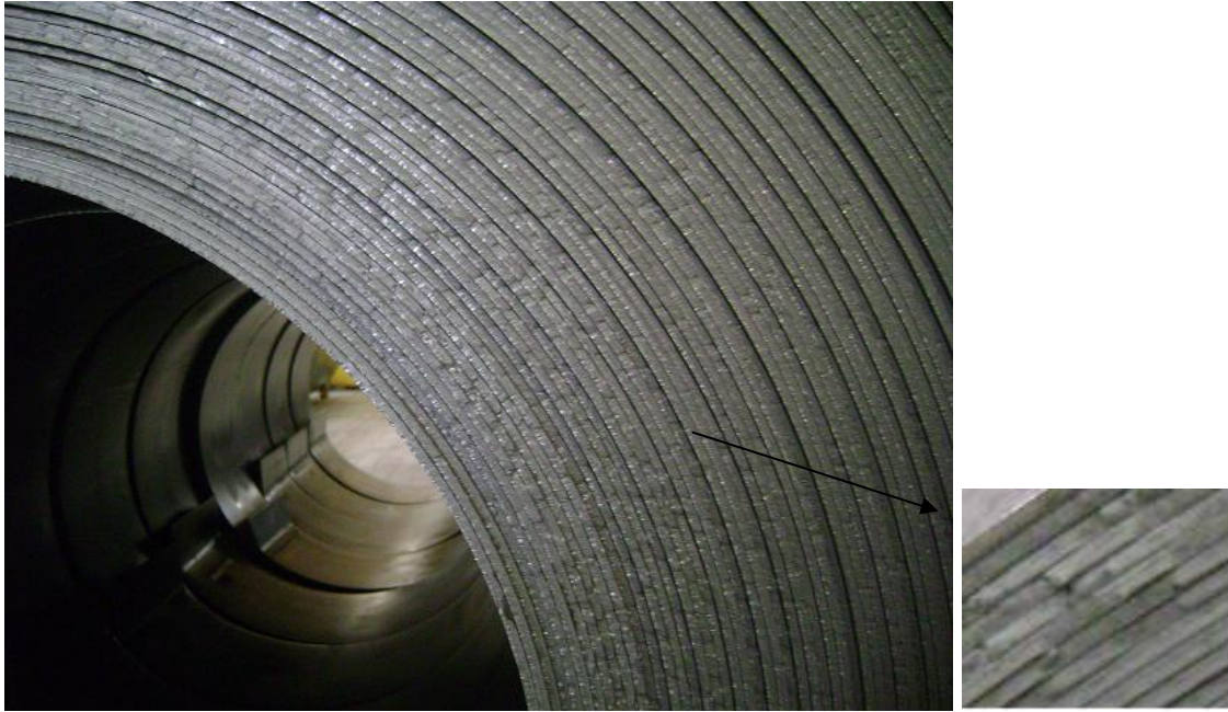
Figura 6 – Corte cisalhado.
