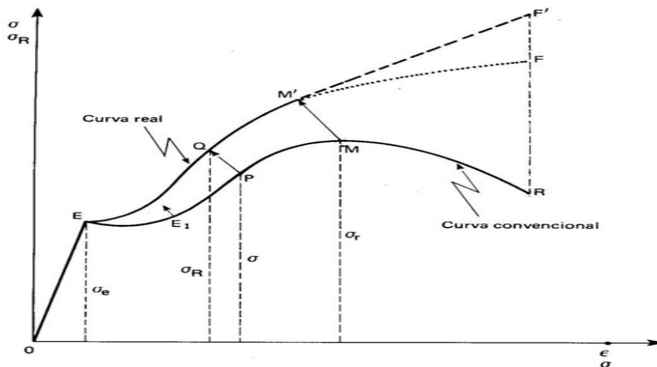
Figura 1 - Curvas tensão de deformação real e convencional. (3)
