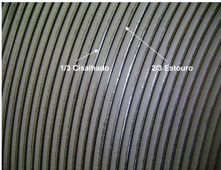
Figura 4 – Corte adequado.
