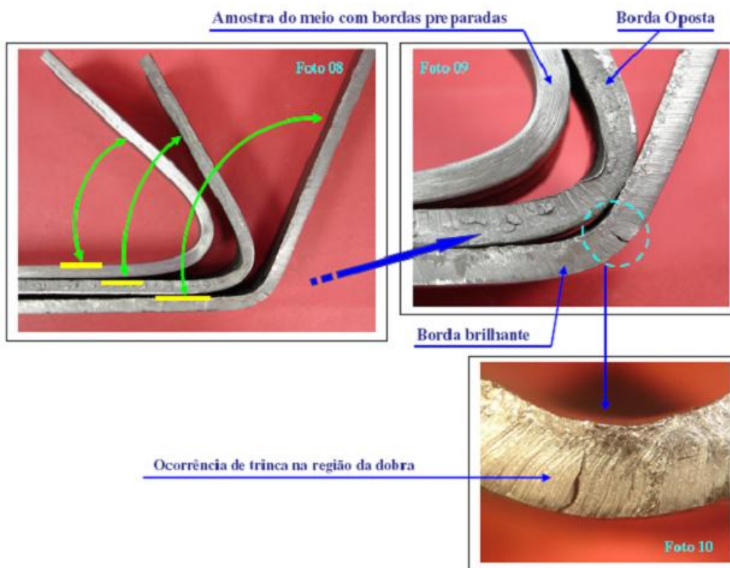
Figura 14 – Teste de dobra.
