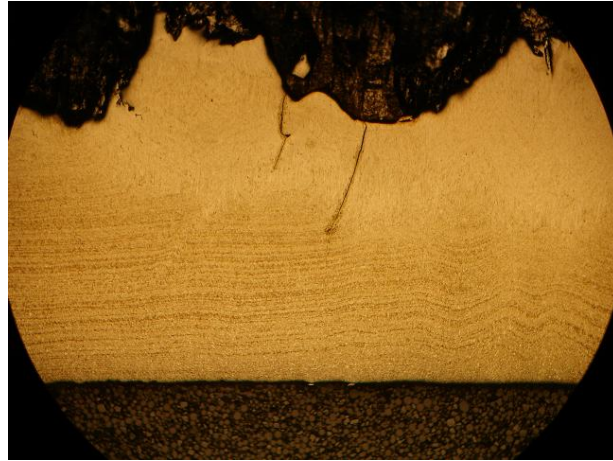
Figura 12 - Microestrutura do corte cisalhado – 100x.
