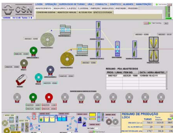
Figura 4. Sinópticos de abastecimento.
