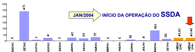
Figura 13. Desvios por corte irregular (t).
