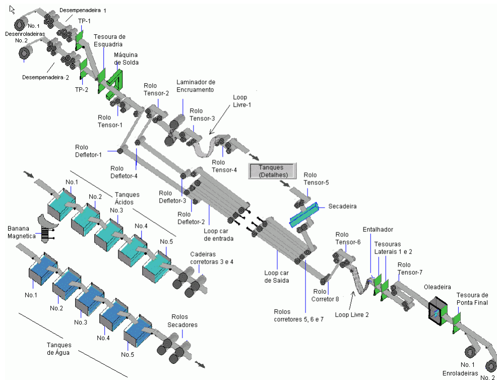
Figura 1. Fluxo do processo de uma Linha de Decapagem Ácida da CSN.
