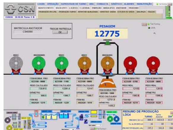
Figura 5. Esteira e balança.
