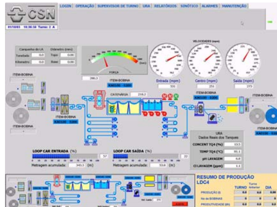
Figura 3. Sinóptico geral da Linha de decapagem 4 da CSN.
