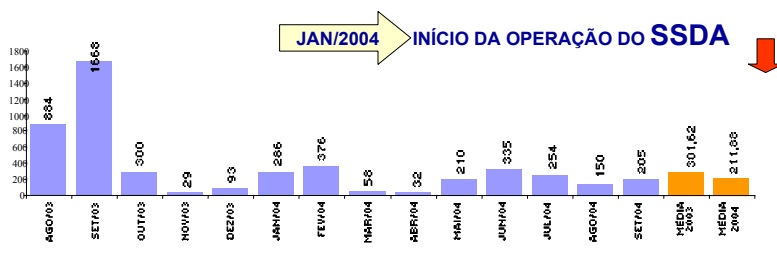
Figura 12. Desvios por serrilhado (t).
