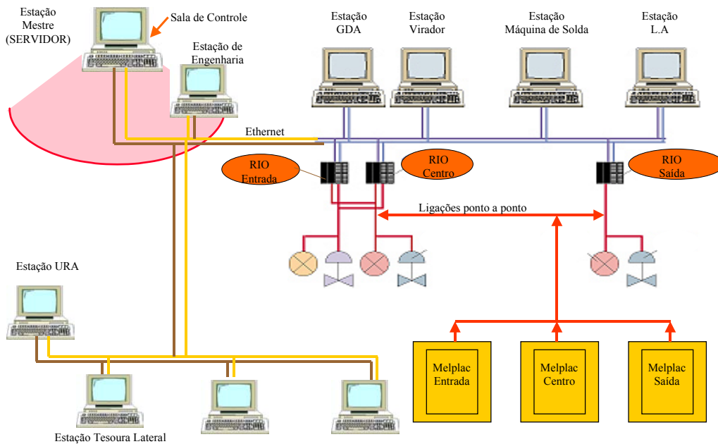
Figura 2. Arquitetura do Sistema SSDA.
