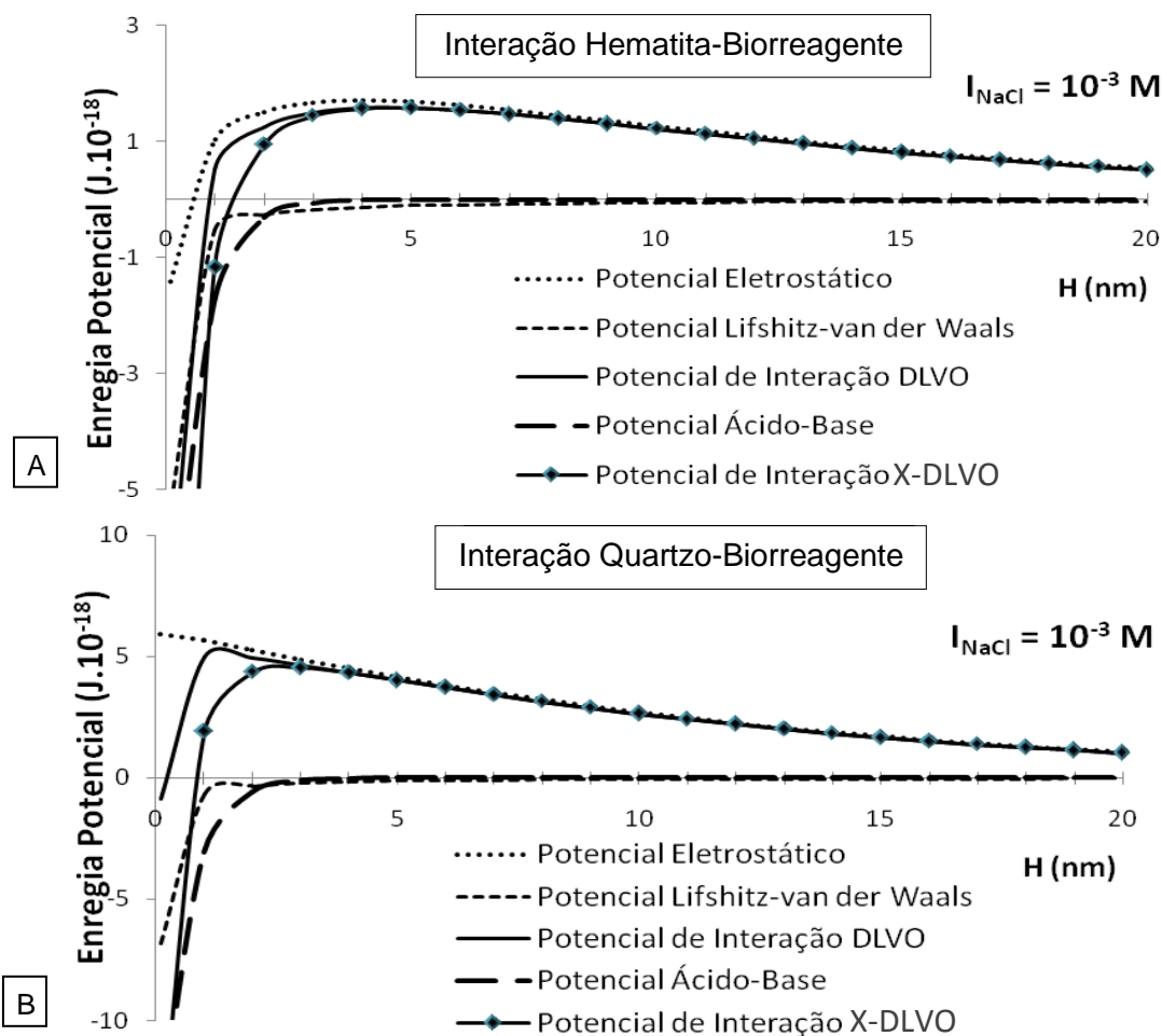
Figura 2. Curva de energia em função da distância para os sistemas hematita-reagente (A) e para o sistema quartzo-reagente (B), ambos em pH 6.
