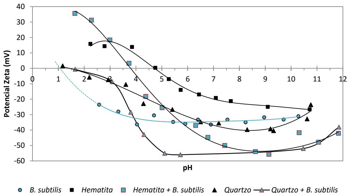
Figura 1. Potencial zeta da hematita antes e após interação com B. subtilis . 1.10^{-3} M NaCl como eletrólito indifferente. Concentração bacteriana 600 \text{ mg.L}^{-1} .
