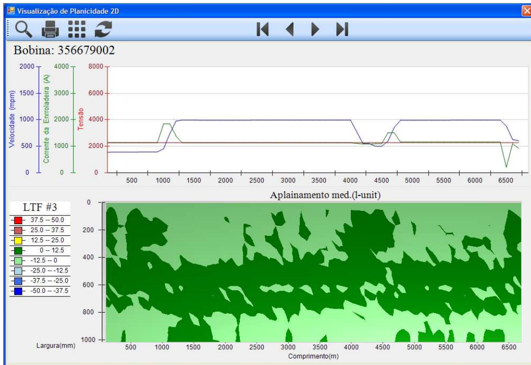
Figura 4 – Tela com o gráfico de aplainamento.
