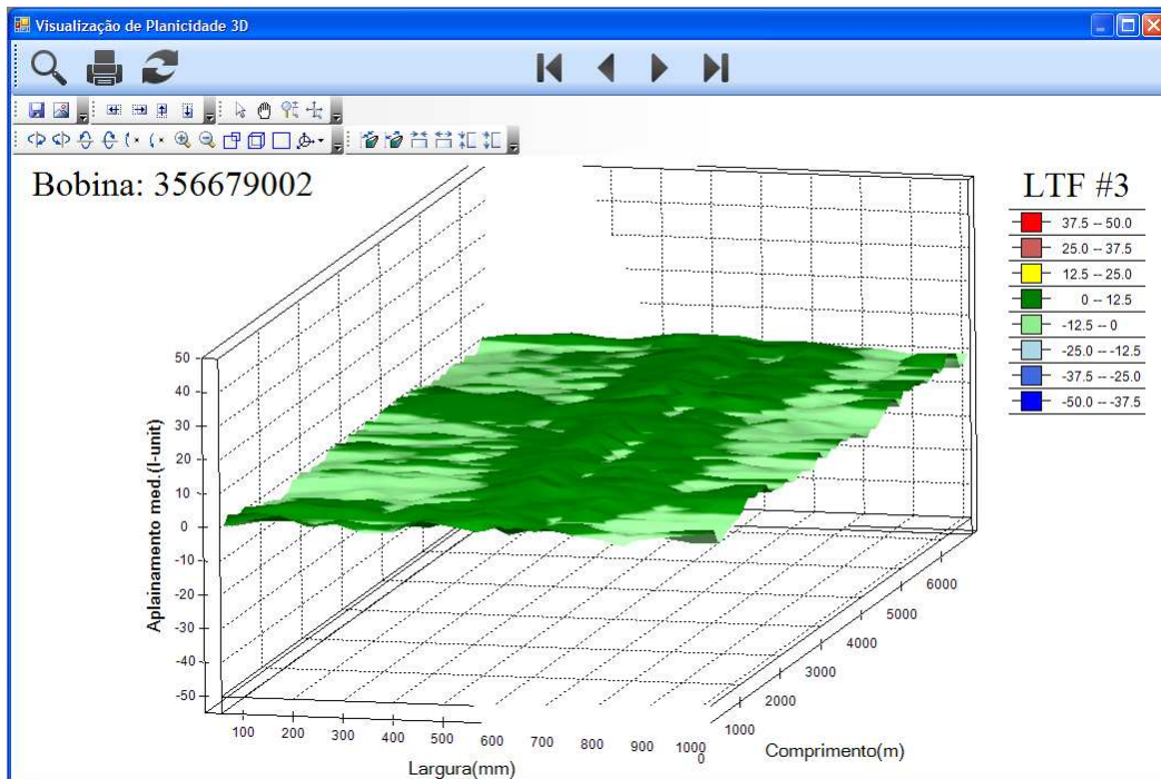
Figura 5 – Tela com o perfil de aplainamento.
