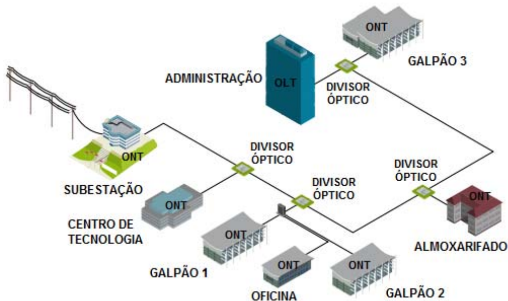
Figura 3 – Exemplo de rede óptica passiva na indústria
