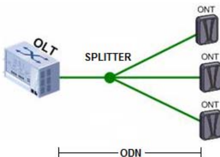
Figura 4 - Elementos de uma rede óptica passiva
