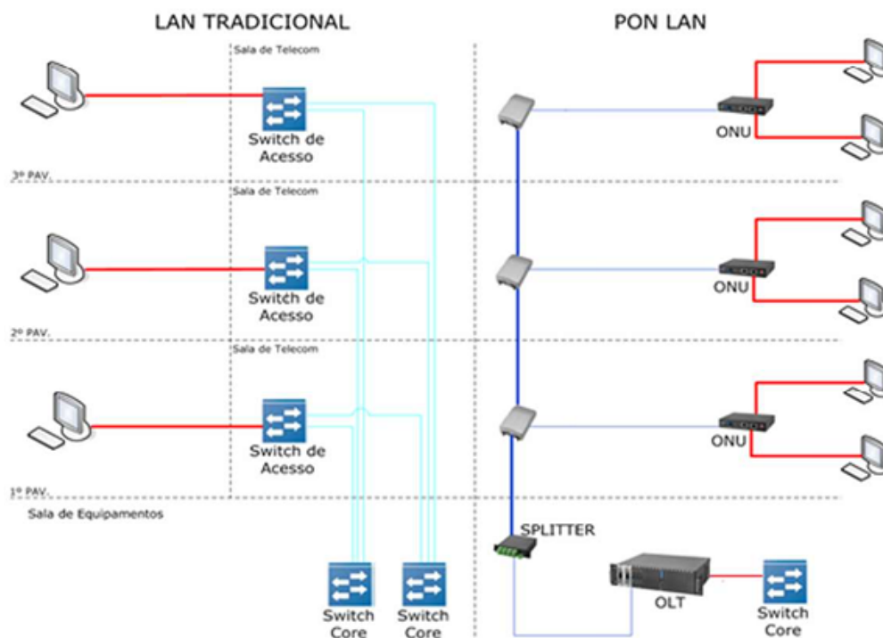
Figura 5 – Simplificação na configuração e no gerenciamento
