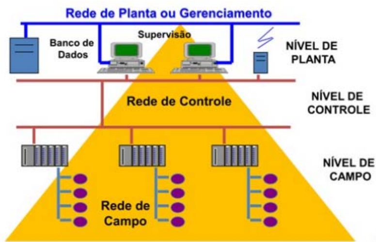
Figura 2 - Rede industrial típica
