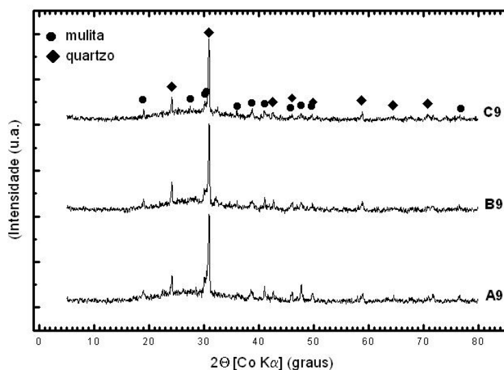
Figura 2. Difratogramas das composições queimadas a 1200°C.
