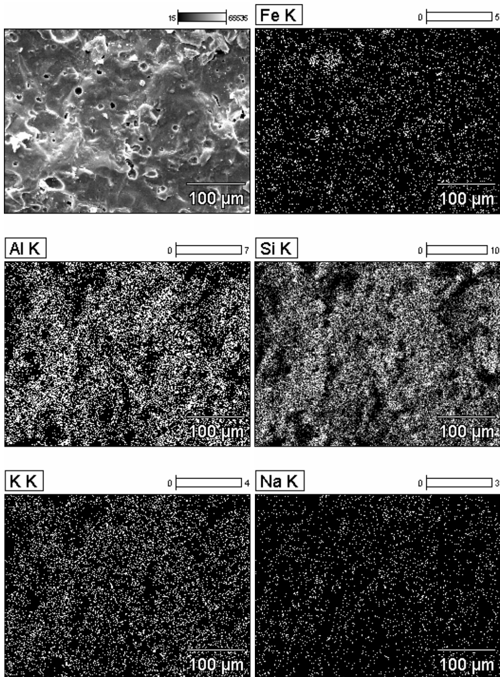
Figura 8. Micrografia obtida por MEV da região de fratura da massa C , queimada a 1200 °C, com mapeamento de elementos químicos por EDS.
