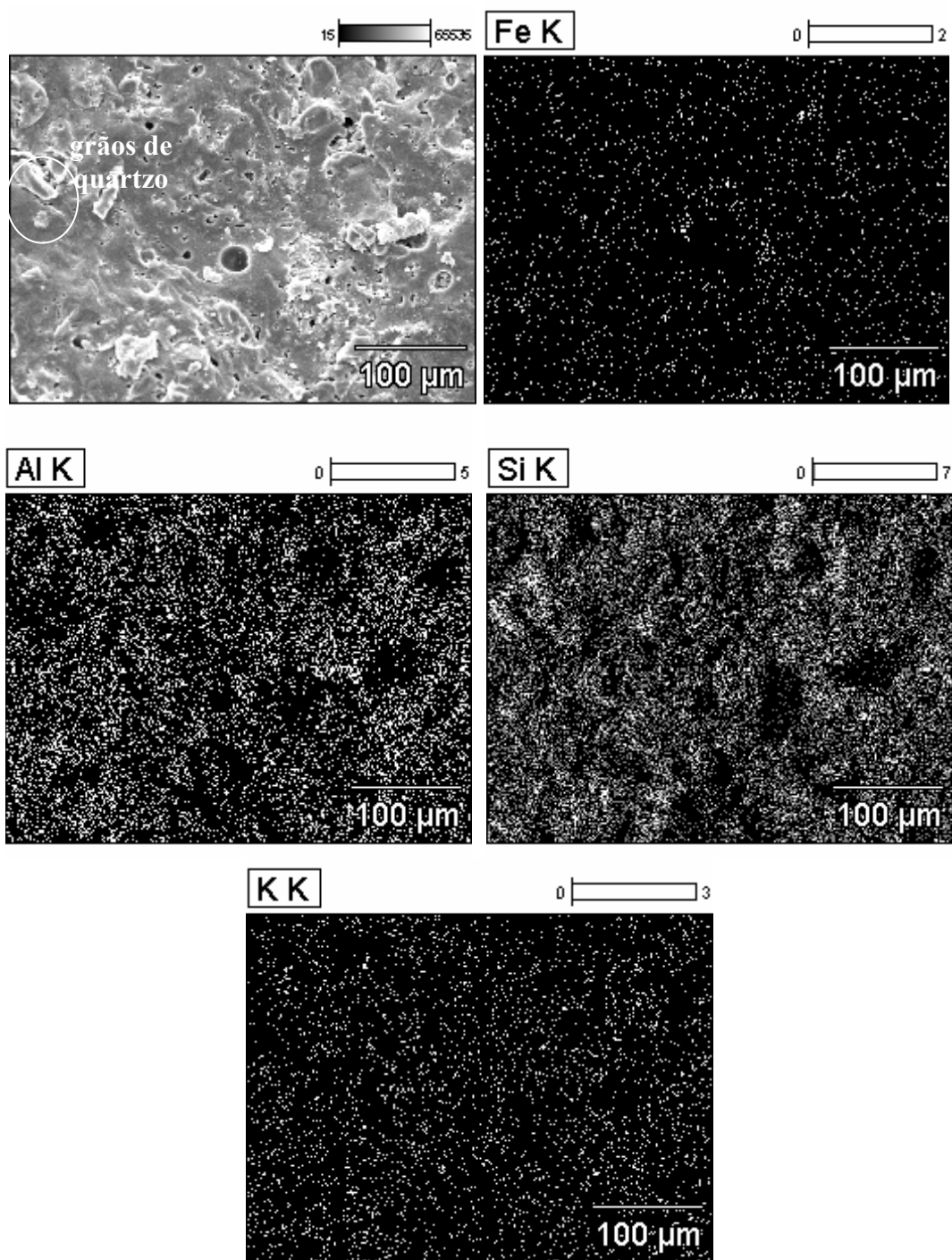
Figura 6. Micrografia obtida por MEV da região de fratura da massa A com mapeamento de elementos químicos por EDS.
