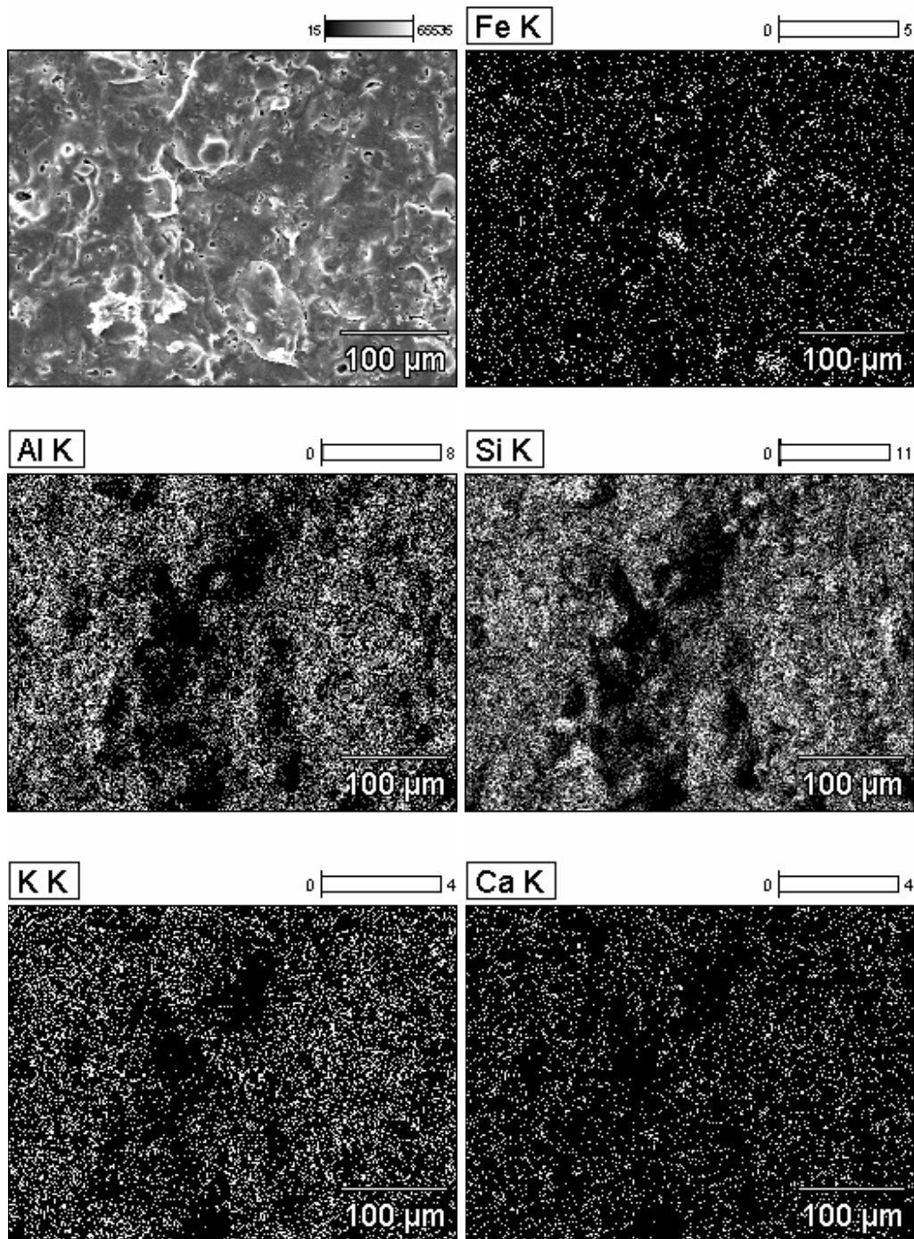
Figura 7. Micrografia obtida por MEV da região de fratura da massa B , queimada a 1200 °C, com mapeamento de elementos químicos por EDS.
